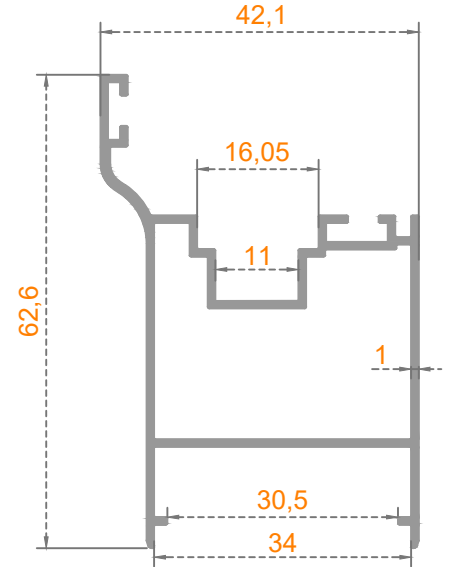
Sistem Kodu: 41-2943 Ağırlık (kg/mt) 0,610
