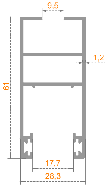
Sistem Kodu: 53-4575 Ağırlık (kg/mt) 0,730
