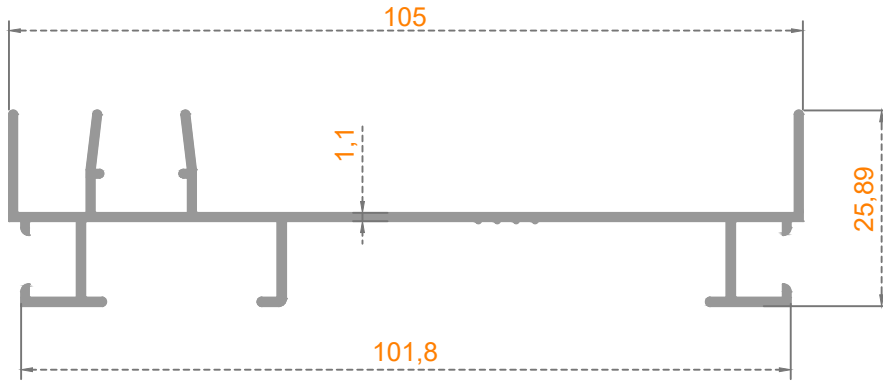
Sistem Kodu: 54-4770 Ağırlık (kg/mt) 0,540
