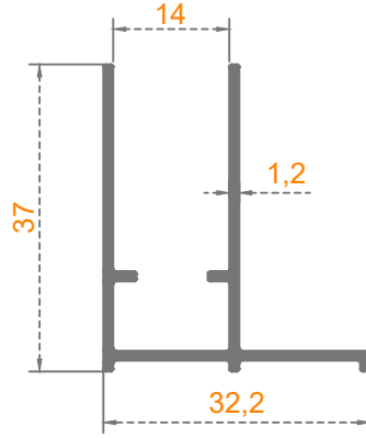
DUVAR DİKMESİ
