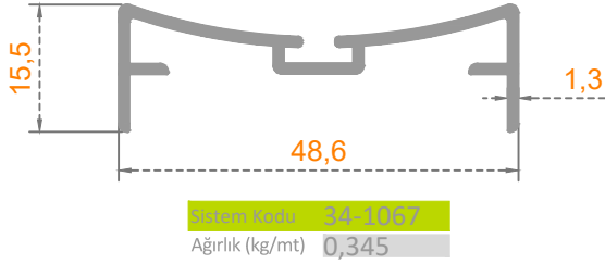
ÇARPMA KAPI İÇ
