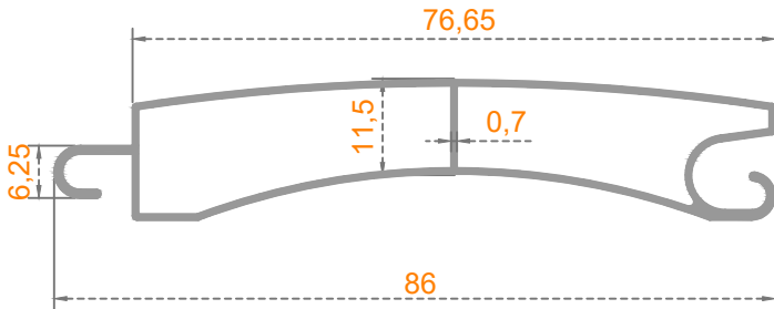
Sistem Kodu: 38-1205 Ağırlık (kg/mt) 0,450
