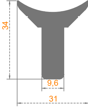
- Y- BAĞLANTI
