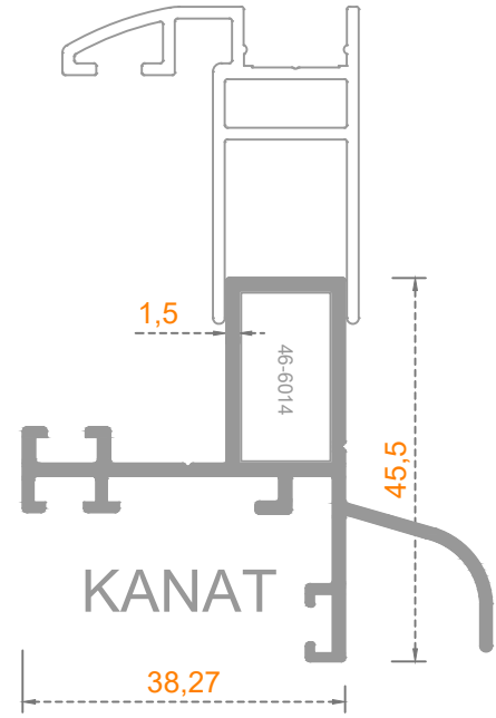
Sistem Kodu: 50-11003 Ağırlık (kg/mt) 0,716
