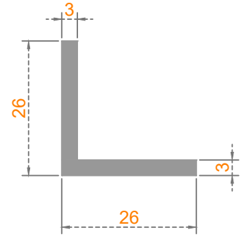
Sistem Kodu: 24-308 Ağırlık (kg/mt) 0,400
