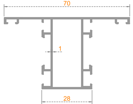
Sistem Kodu: 53-4505 Ağırlık (kg/mt) 0,730
