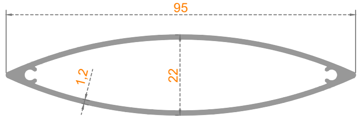
GÜNEŞ KIRICI
