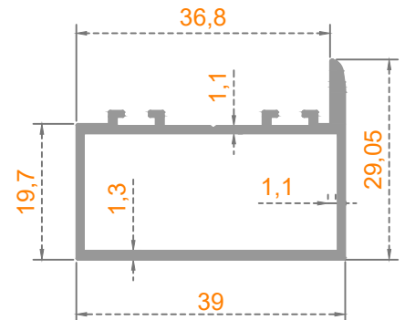
Sistem Kodu: 41-2783 Ağırlık (kg/mt) 0,451
