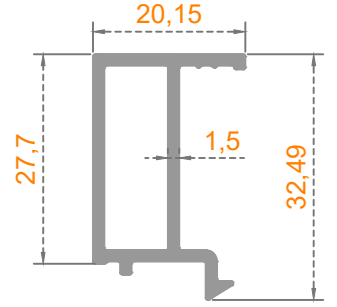
Sistem Kodu: 54-4779 Ağırlık (kg/mt) 0,386
