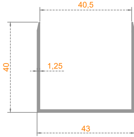
Sistem Kodu: 41-2913 Ağırlık (kg/mt) 0,406
