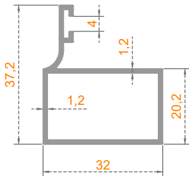
Sistem Kodu: 41-2386 Ağırlık (kg/mt) 0,420
