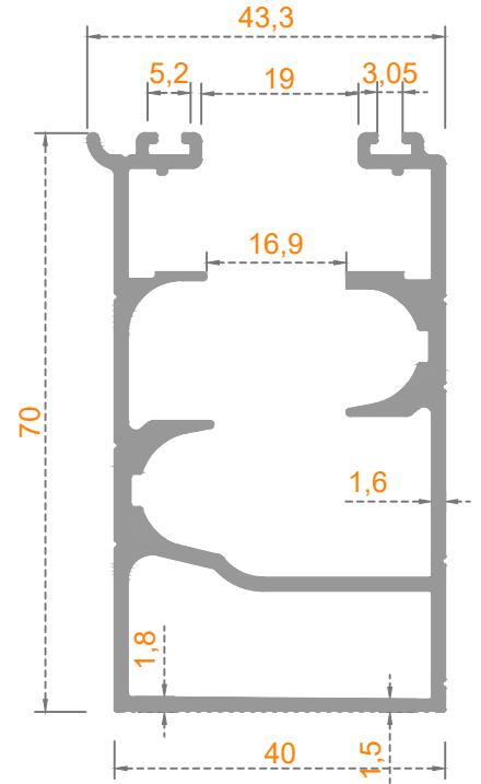
Sistem Kodu: 41-2849 Ağırlık (kg/mt) 1,375
