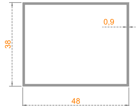
Sistem Kodu: 20-133 Ağırlık (kg/mt) 0,415
