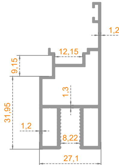
Sistem Kodu: 41-2933 Ağırlık (kg/mt) 0,755
