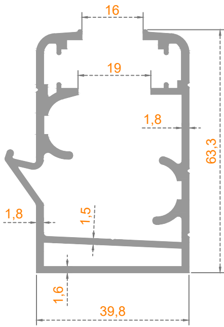
Sistem Kodu: 41-2451 Ağırlık (kg/mt) 1,365
