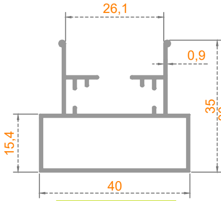
Sistem Kodu: 40-1313-0 Ağırlık (kg/mt) 0,440
