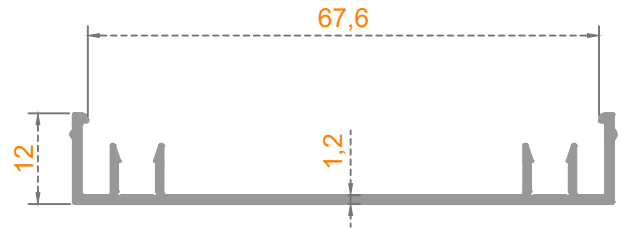
Sistem Kodu: 50-1635 Ağırlık (kg/mt) 0,379
