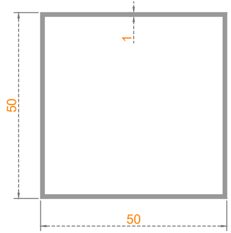
Sistem Kodu: 20-146 Ağırlık (kg/mt) 0,535
