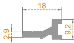
Sistem Kodu: 50-1620 Ağırlık (kg/mt) 0,195
