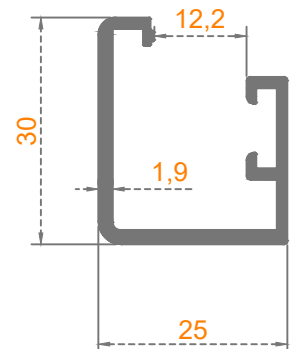
Sistem Kodu: 58-2280 Ağırlık (kg/mt) 0,420
