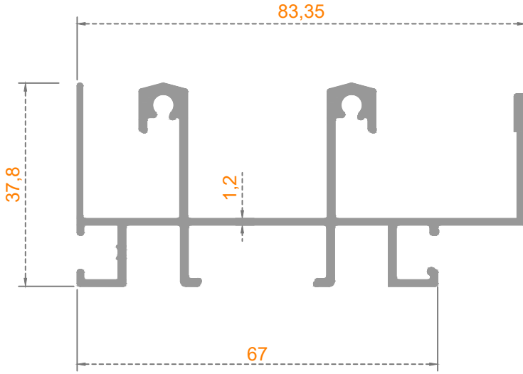
Sistem Kodu: 54-4730 Ağırlık (kg/mt) 1,063
