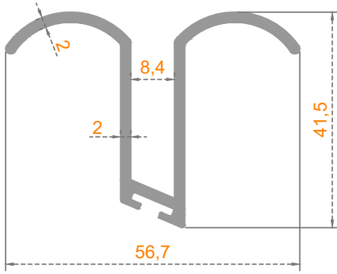
Sistem Kodu: 41-2787 Ağırlık (kg/mt) 0,715
