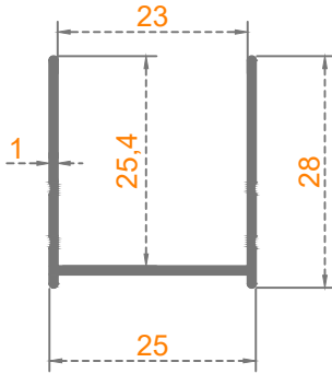
GENİŞ DUVAR DİKMESİ
