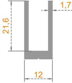
SÜRME - U -
