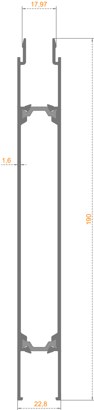
Sistem Kodu: 66-1311 Ağırlık (kg/mt) 2,111
