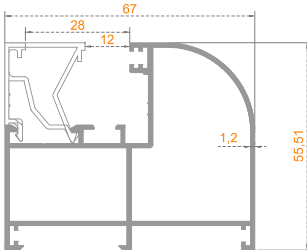
Sistem Kodu: 49-4305 Ağırlık (kg/mt) 1,000
