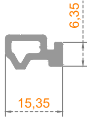
Sistem Kodu: 50-1489 Ağırlık (kg/mt) 0,190
