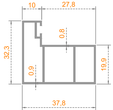
Sistem Kodu: 41-2344 Ağırlık (kg/mt) 0,415
