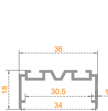
Sistem Kodu: 41-2940 Ağırlık (kg/mt) 0,265
