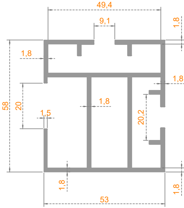
Sistem Kodu 30-523 Ağırlık (kg/mt) 1,590
