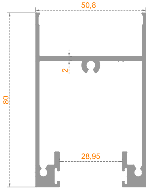
Sistem Kodu: 54-4794 Ağırlık (kg/mt) 1,332
