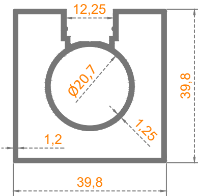
Sistem Kodu: 58-2222 Ağırlık (kg/mt) 0,770
