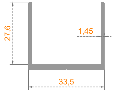
GENİŞ - U - (IRAK İÇİN)
