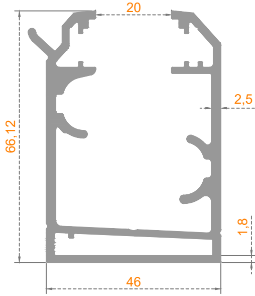
Sistem Kodu: 41-2702 Ağırlık (kg/mt) 1,741
