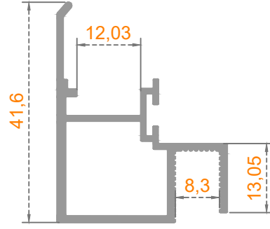
Sistem Kodu: 80-5259 Ağırlık (kg/mt) 0,486
