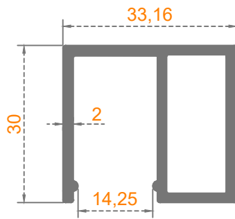
Sistem Kodu: 58-2269 Ağırlık (kg/mt) 0,680
