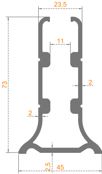
Sistem Kodu: 58-2211 Ağırlık (kg/mt) 1,490
