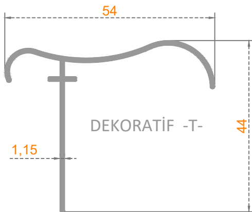
Sistem Kodu: 26-403 Ağırlık (kg/mt) 0,360
