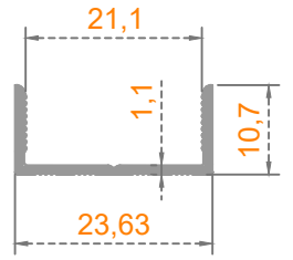
Sistem Kodu: 48-4256 Ağırlık (kg/mt) 0,130
