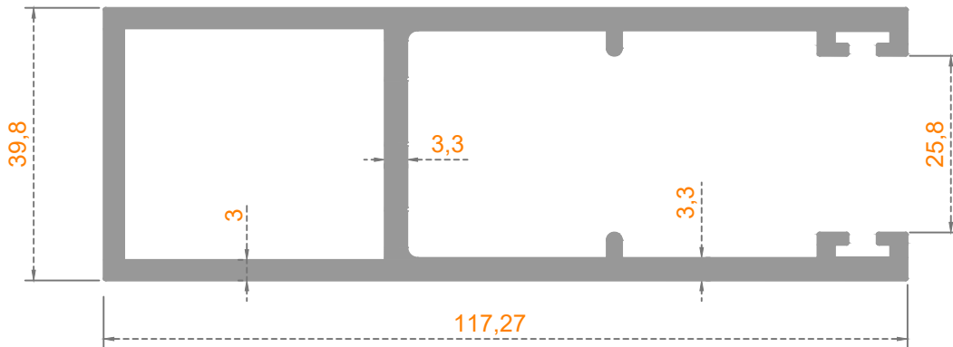
Sistem Kodu: 38-1229 Ağırlık (kg/mt) 2,800
