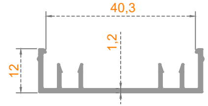
Sistem Kodu: 50-1625 Ağırlık (kg/mt) 0,292
