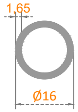
Sistem Kodu: 22-218 Ağırlık (kg/mt) 0,205
