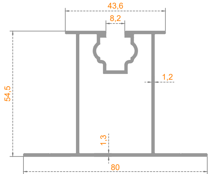
Sistem Kodu 80-5201 Ağırlık (kg/mt) 0,915
