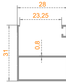
Sistem Kodu: 40-1331 Ağırlık (kg/mt) 0,265
