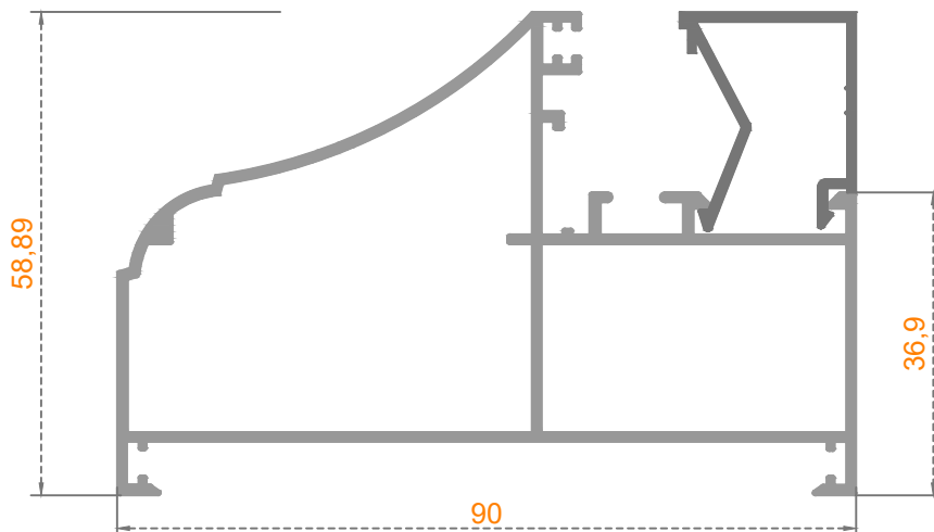
Sistem Kodu: 49-4411 Ağırlık (kg/mt) 1,181
