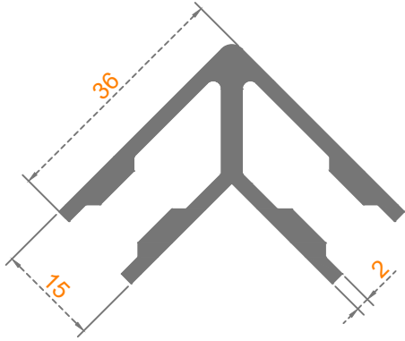
ALDOKS DAR ÇAVUŞ
