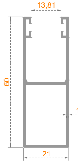
Sistem Kodu: 38-1242 Ağırlık (kg/mt) 0,487
