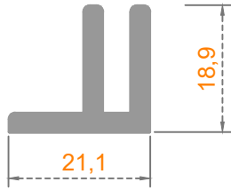
Sistem Kodu: 50-1658 Ağırlık (kg/mt) 0,435
