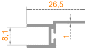
Sistem Kodu: 41-2393 Ağırlık (kg/mt) 0,156
