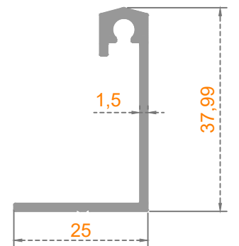
Sistem Kodu: 54-4834 Ağırlık (kg/mt) 0,350
