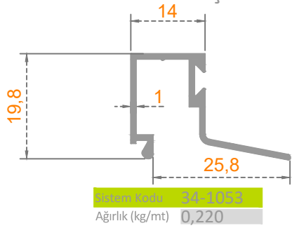
TEK CAM CONTASIZ ÇITA
