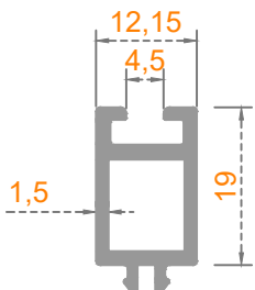
Sistem Kodu: 50-1608 Ağırlık (kg/mt) 0,285
