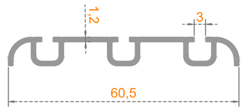
Profil Kodu: 41-2767 Ağırlık (kg/mt) 0,365
