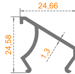
Sistem Kodu: 58-2389 Ağırlık (kg/mt) 0,230
