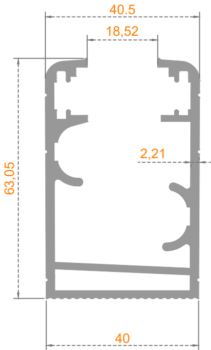
Sistem Kodu 41-2462 Ağırlık (kg/mt) 1,471
