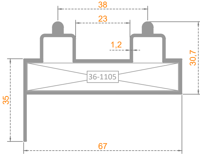
KULAKLI RAYLI KASA
