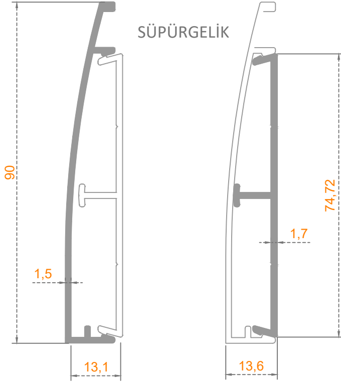
Sistem Kodu: 48-4219 Ağırlık (kg/mt) 0,480
