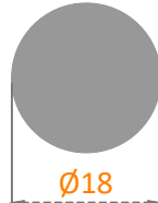
Sistem Kodu: 22-252 Ağırlık (kg/mt) 0,690
