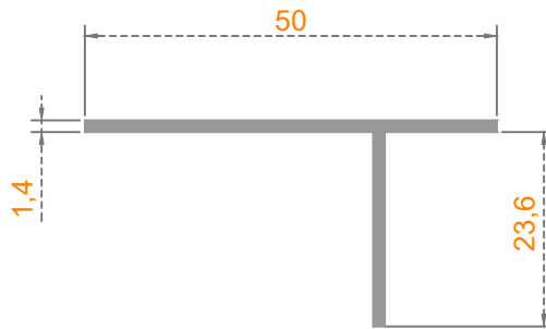
Sistem Kodu: 26-402 Ağırlık (kg/mt) 0,280
