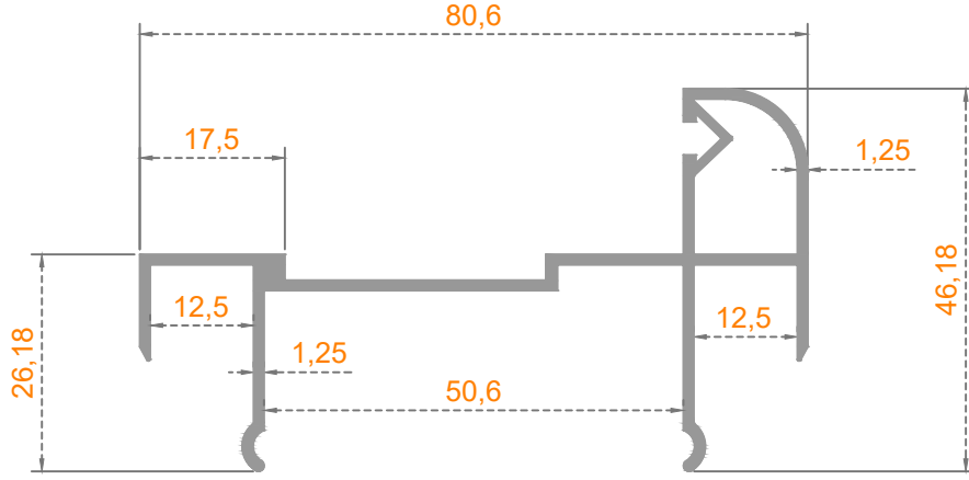
Sistem Kodu: 39-1273 Ağırlık (kg/mt) 0,740
