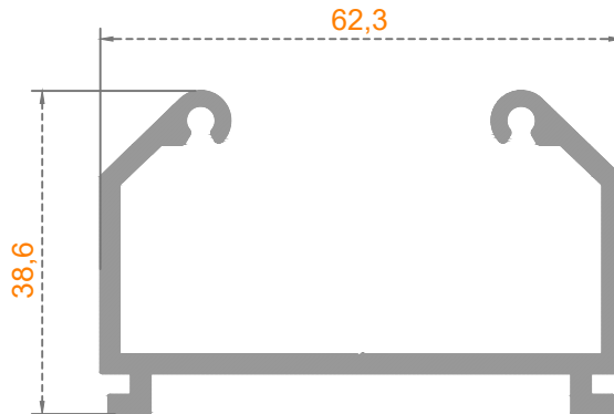
Sistem Kodu: 54-4843 Ağırlık (kg/mt) 1,005
