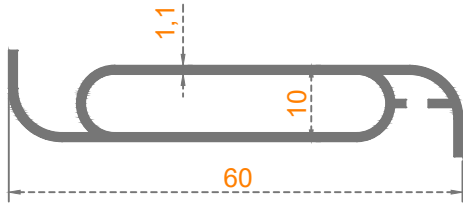
LÜKS MENFEZ KANAT
