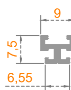
Sistem Kodu: 48-4241 Ağırlık (kg/mt) 0,085
