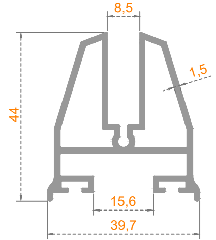
Sistem Kodu: 41-2712 Ağırlık (kg/mt) 0,855
