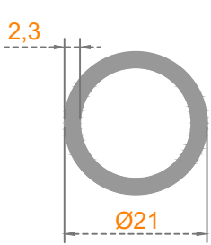
Sistem Kodu: 22-245 Ağırlık (kg/mt) 0,370
