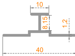
Sistem Kodu: 26-418 Ağırlık (kg/mt) 0,207
