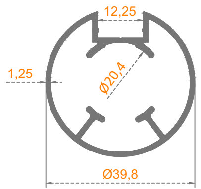
Ø 40'LIK DİKME
