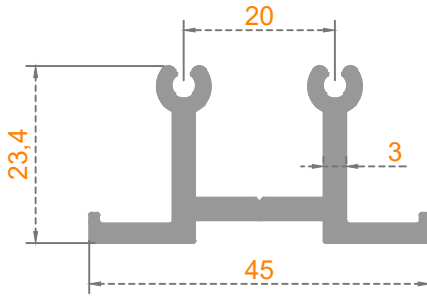
Sistem Kodu: 50-1631 Ağırlık (kg/mt) 0,730
