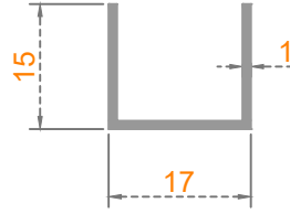
Sistem Kodu: 38-1201 Ağırlık (kg/mt) 0,125
