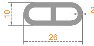
Sistem Kodu: 48-4248 Ağırlık (kg/mt) 0,345
