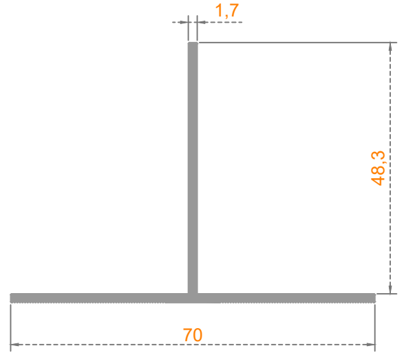
Sistem Kodu: 26-407 Ağırlık (kg/mt) 0,525
