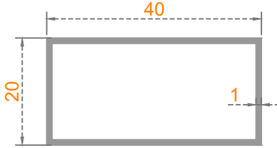
Sistem Kodu: 20-161 Ağırlık (kg/mt) 0,315
