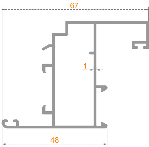
Sistem Kodu: 53-4561 Ağırlık (kg/mt) 0,670
