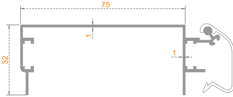
ÖZEL KASA
