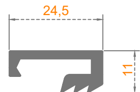
Sistem Kodu: 56-1508 Ağırlık (kg/mt) 0,315
