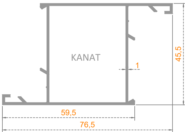
Sistem Kodu: 32-1005 Ağırlık (kg/mt) 0,660
