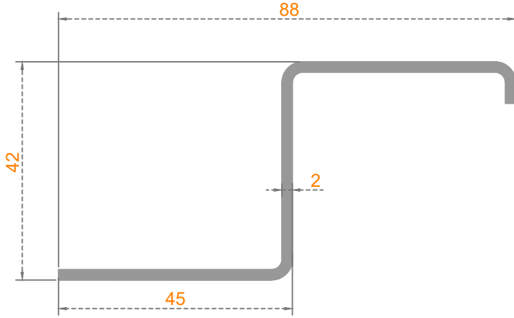
Sistem Kodu: 50-1052 Ağırlık (kg/mt) 0,730
