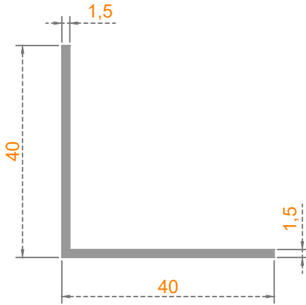
Sistem Kodu: 24-313 Ağırlık (kg/mt) 0,325
