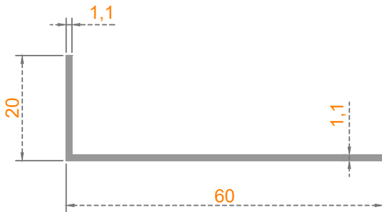
Sistem Kodu: 24-319 Ağırlık (kg/mt) 0,245
