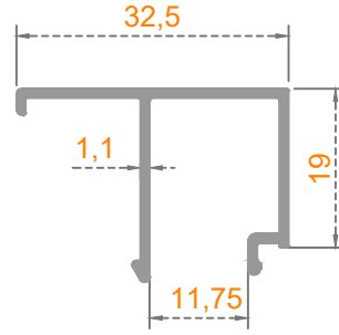
10 MM ÇITA
