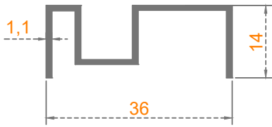
LÜKS MENFEZ KAPAK
