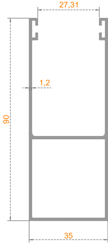
Sistem Kodu: 38-1244 Ağırlık (kg/mt) 0,855
