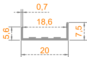
Sistem Kodu: 48-4238 Ağırlık (kg/mt) 0,070
