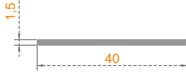
Sistem Kodu: 41-2325 Ağırlık (kg/mt) 0,170
