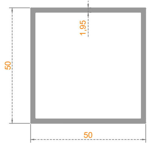
Sistem Kodu: 20-133 Ağırlık (kg/mt) 1,010
