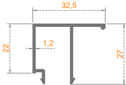
KASA TEK CAM ÇITA
