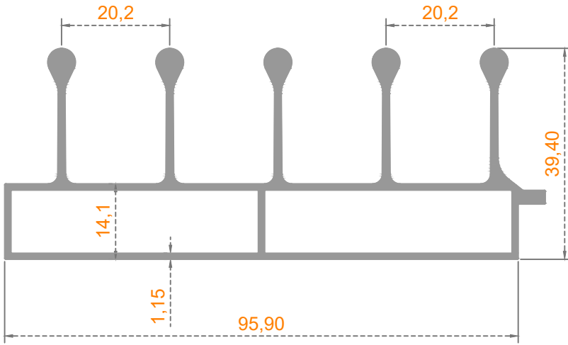
Profil Kodu: 41-2911 Ağırlık (kg/mt) 1,490
