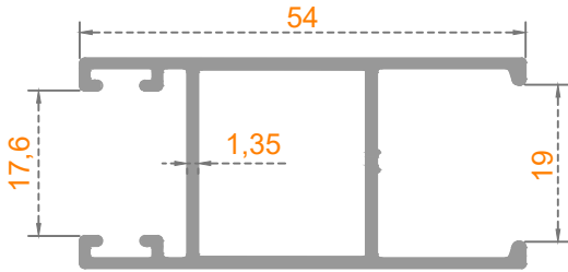
Sistem Kodu: 54-4732 Ağırlık (kg/mt) 0,610
