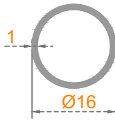
Sistem Kodu: 22-258 Ağırlık (kg/mt) 0,130
