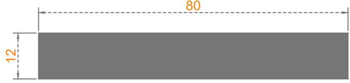
Sistem Kodu: 58-2275 Ağırlık (kg/mt) 2,605
