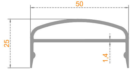
Sistem Kodu: 50-1054 Ağırlık (kg/mt) 0,512
