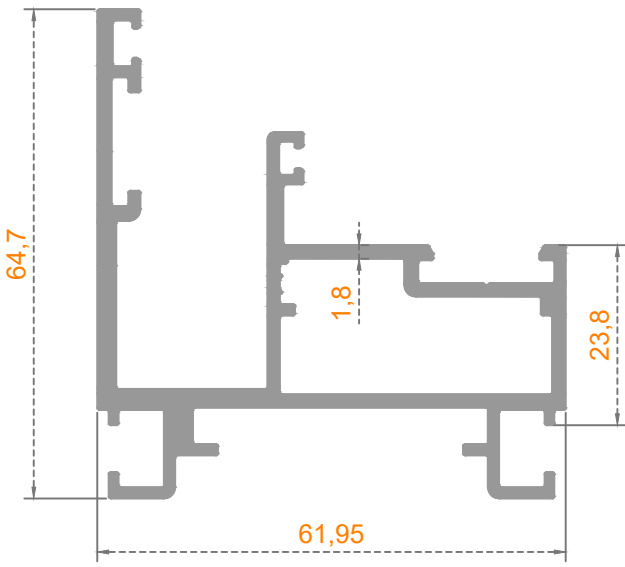
Sistem Kodu: 54-4796 Ağırlık (kg/mt) 1,505
