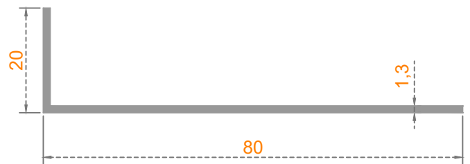
Sistem Kodu: 24-310 Ağırlık (kg/mt) 0,355
