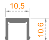
Sistem Kodu: 58-2207 Ağırlık (kg/mt) 0,105
