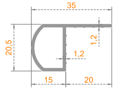
Sistem Kodu: 48-4235-1 Ağırlık (kg/mt) 0,263
