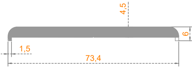
Sistem Kodu: 58-2260 Ağırlık (kg/mt) 0,910
