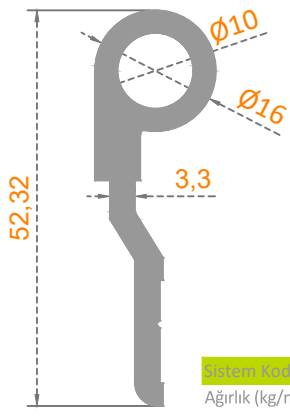
ALDOKS DÜZ KASA MENTEŞE
