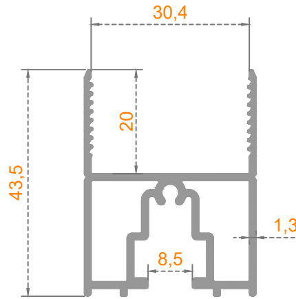
Sistem Kodu: 41-2929 Ağırlık (kg/mt) 0,679
