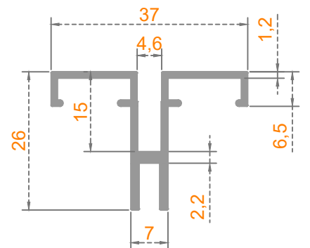
Sistem Kodu: 48-4242 Ağırlık (kg/mt) 0,375
