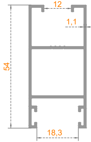
Sistem Kodu: 54-4772 Ağırlık (kg/mt) 0,554
