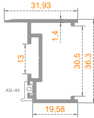
Sistem Kodu: 41-2878 Ağırlık (kg/mt) 0,393
