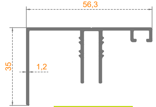
Sistem Kodu: 66-1307 Ağırlık (kg/mt) 0,525
