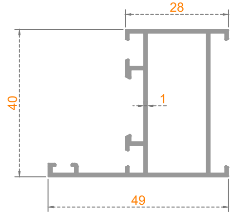
Sistem Kodu: 53-4503 Ağırlık (kg/mt) 0,507
