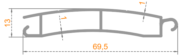
Sistem Kodu: 38-1220 Ağırlık (kg/mt) 0,465
