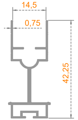
Sistem Kodu: 40-1328 Ağırlık (kg/mt) 0,295
