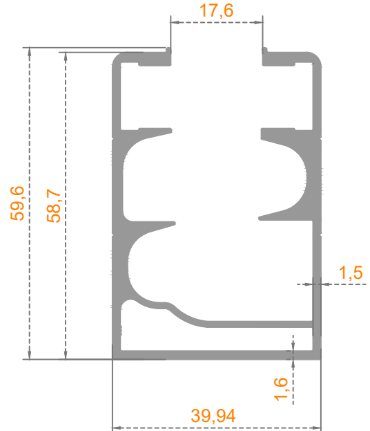
Sistem Kodu: 41-2948 Ağırlık (kg/mt) 1,248
