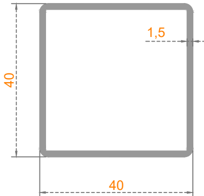
Sistem Kodu: 20-132 Ağırlık (kg/mt) 0,625
