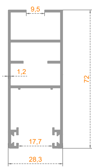
Sistem Kodu: 53-4581 Ağırlık (kg/mt) 0,845
