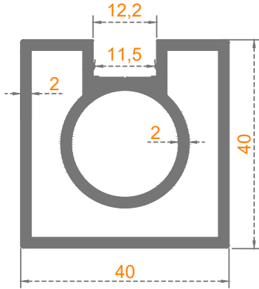
Sistem Kodu: 58-2261 Ağırlık (kg/mt) 1,265
