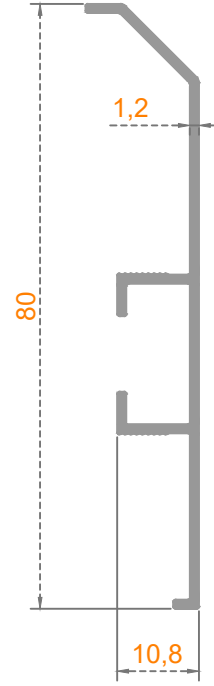
Sistem Kodu: 48-4255 Ağırlık (kg/mt) 0,390
