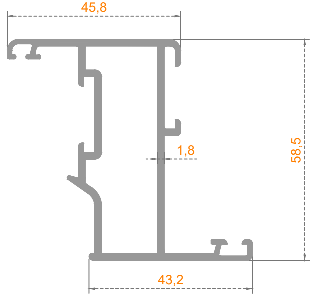
Sistem Kodu: 55-2127 Ağırlık (kg/mt) 1,135
