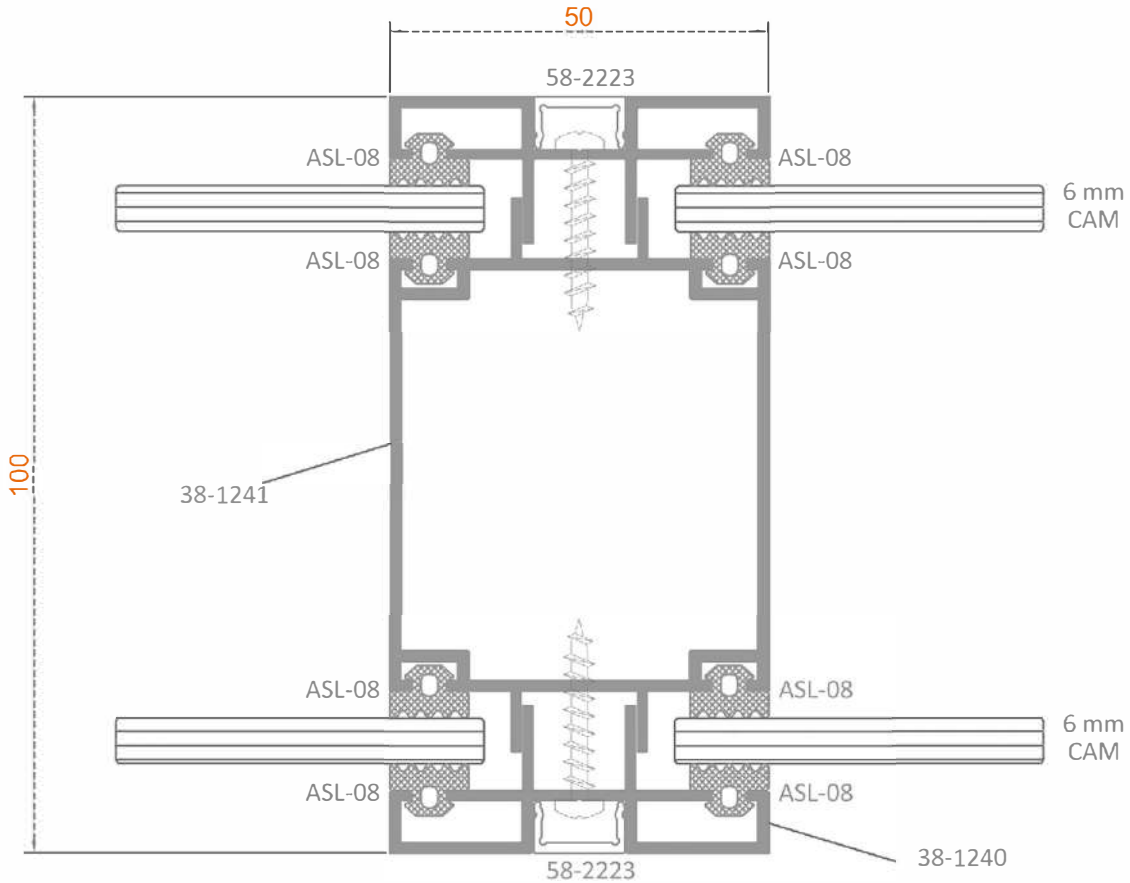
Sistem Kodu: 38-1241 Ağırlık (kg/mt) 1,005
