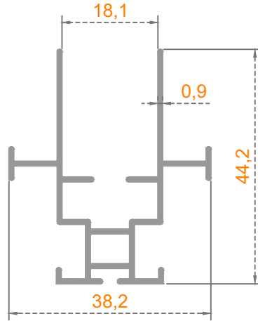
Sistem Kodu: 40-1314-C Ağırlık (kg/mt) 0,425
