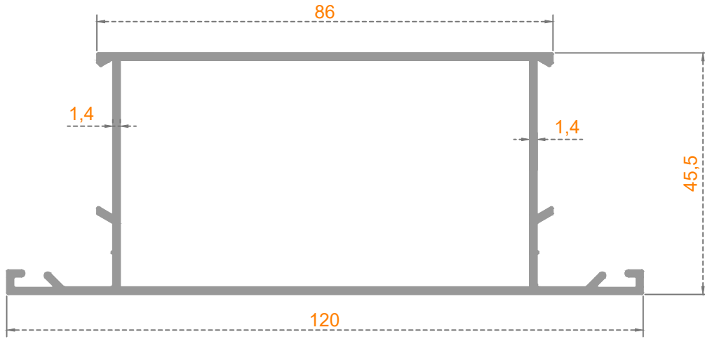
Sistem Kodu: 32-1007 Ağırlık (kg/mt) 1,200
