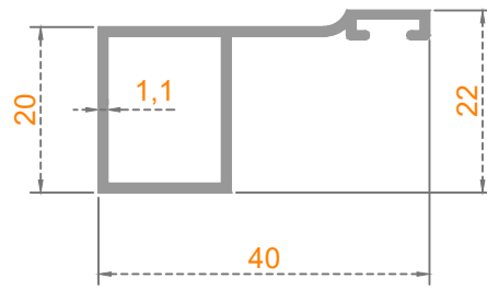
Sistem Kodu: 40-1310 Ağırlık (kg/mt) 0,295
