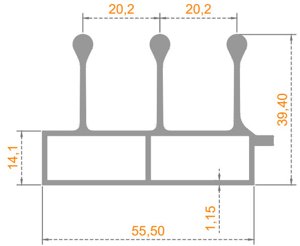
Profil Kodu: 41-2768 Ağırlık (kg/mt) 0,945
