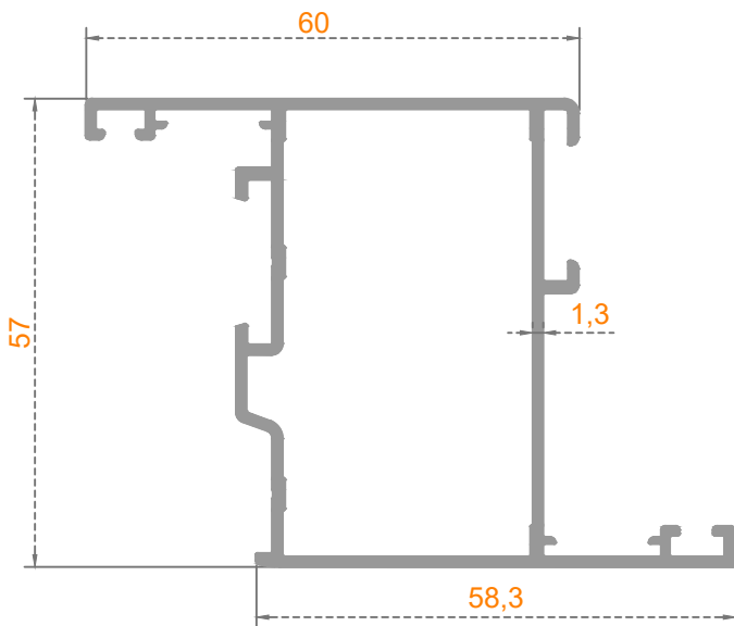
PENCERE KANADI (DÜZ)
