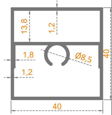
Sistem Kodu: 58-2256 Ağırlık (kg/mt) 0,750
