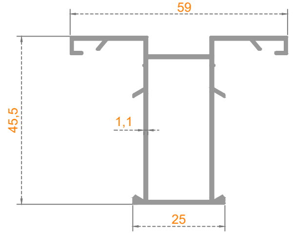
ORTA KAYIT
