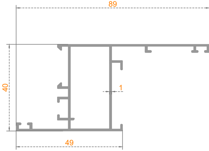
Sistem Kodu: 53-4562 Ağırlık (kg/mt) 0,665
