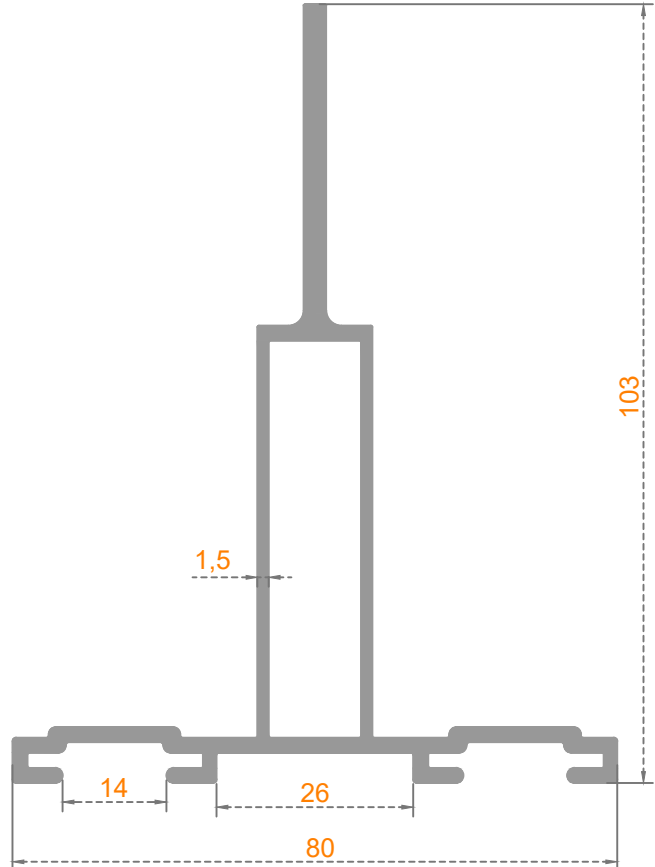
Sistem Kodu: 50-1660 Ağırlık (kg/mt) 1,510
