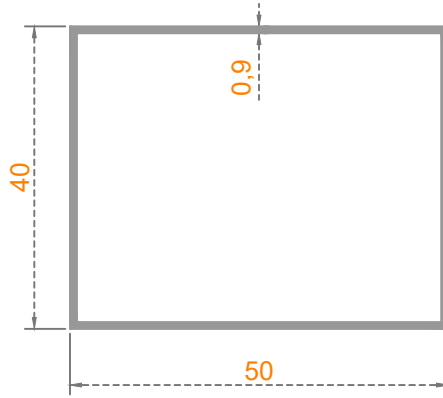
Sistem Kodu: 20-104 Ağırlık (kg/mt) 0,440
