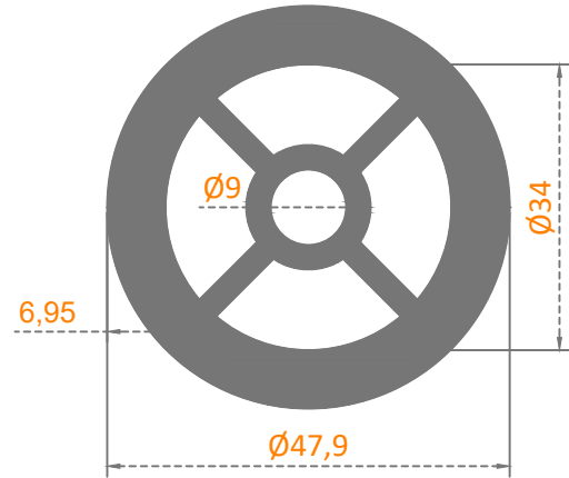
Sistem Kodu: 58-2231 Ağırlık (kg/mt) 3,010
