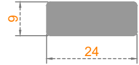
Sistem Kodu: 38-1216 Ağırlık (kg/mt) 0,585
