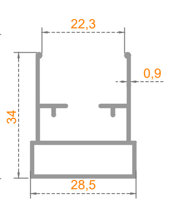
Sistem Kodu: 40-1315 Ağırlık (kg/mt) 0,355
