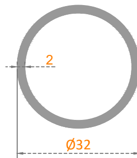
Sistem Kodu: 22-215 Ağırlık (kg/mt) 0,520
