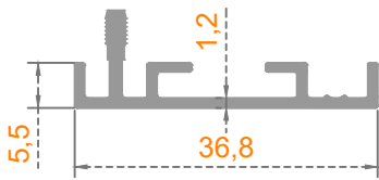
Sistem Kodu: 54-4783 Ağırlık (kg/mt) 0,253
