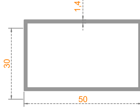
Sistem Kodu: 20-150 Ağırlık (kg/mt) 0,590
