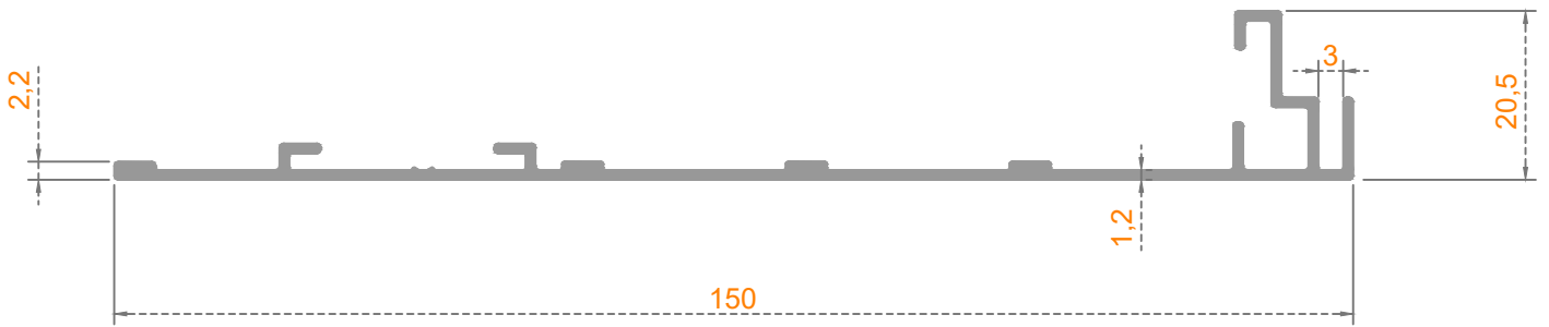
Sistem Kodu: 54-4748 Ağırlık (kg/mt) 0,835
