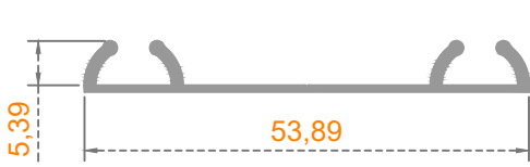
Sistem Kodu: 48-4237 Ağırlık (kg/mt) 0,215
