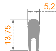
SÜRME RAY
