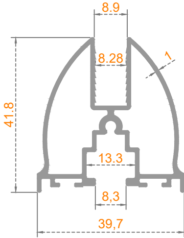
Sistem Kodu: 41-2718 Ağırlık (kg/mt) 0,665
