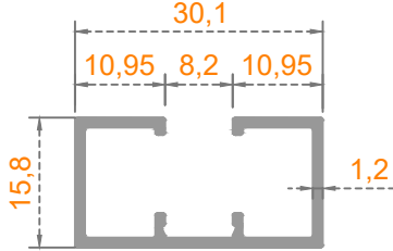
Sistem Kodu: 41-2885 Ağırlık (kg/mt) 0,280
