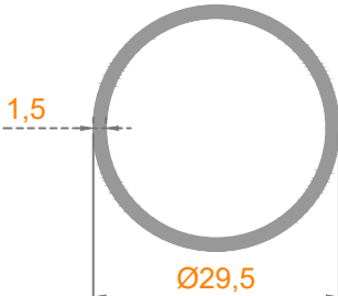
Sistem Kodu: 22-230 Ağırlık (kg/mt) 0,360
