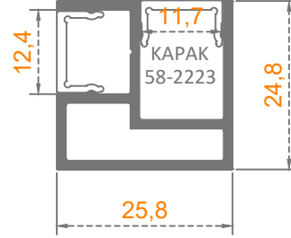
Sistem Kodu: 58-2223 Ağırlık (kg/mt) 0,395
