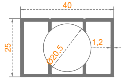
Sistem Kodu: 58-2368 Ağırlık (kg/mt) 0,465
