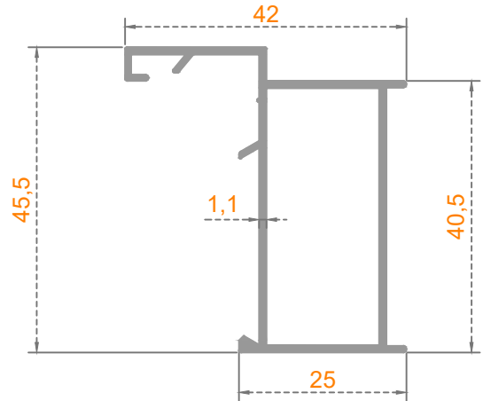
KASA
