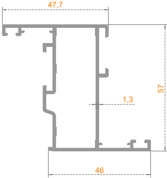
Sistem Kodu: 55-2101 Ağırlık (kg/mt) 0,905
