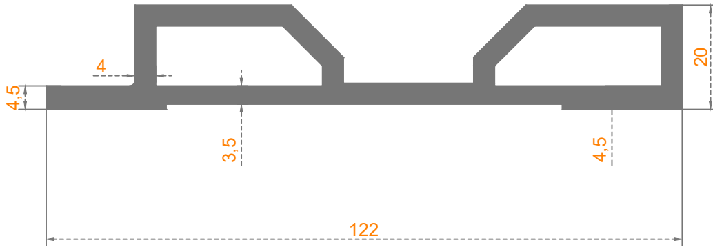
İSKELE PROFİLLER
