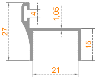
Sistem Kodu: 41-2706 Ağırlık (kg/mt) 0,241
