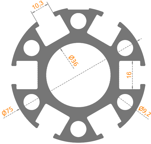
Sistem Kodu: 80-5067 Ağırlık (kg/mt) 4,500
