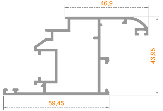
Sistem Kodu: 49-4413 Ağırlık (kg/mt) 0,960
