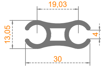
Sistem Kodu: 57-2526 Ağırlık (kg/mt) 0,420
