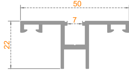
Sistem Kodu: 50-1605 Ağırlık (kg/mt) 0,473
