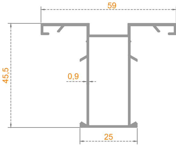
ORTA KAYIT
