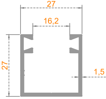
Sistem Kodu: 54-4709 Ağırlık (kg/mt) 0,395
