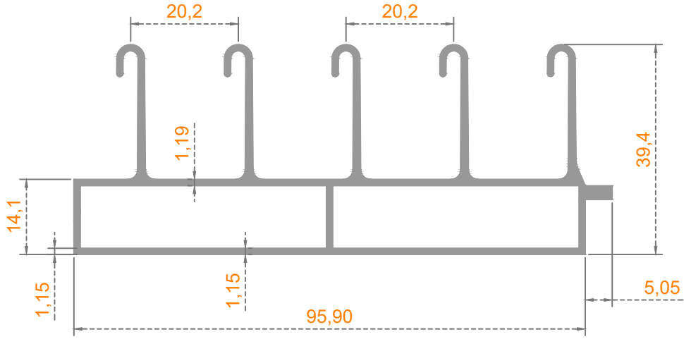
Profil Kodu: 41-2373 Ağırlık (kg/mt) 1,350
