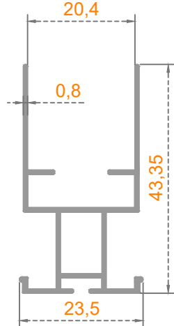
Sistem Kodu: 40-1322 Ağırlık (kg/mt) 0,332
