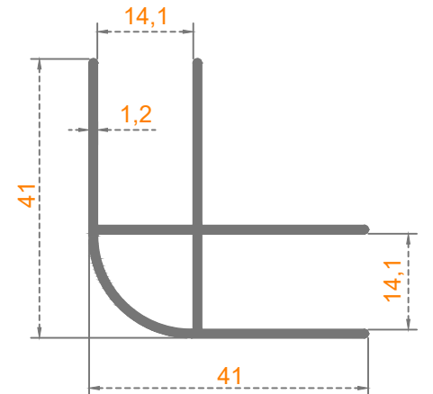
KÖŞE DÖNÜŞ
