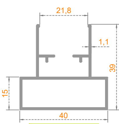
Sistem Kodu: 40-1312 Ağırlık (kg/mt) 0,520
