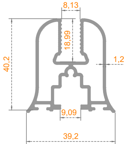
Sistem Kodu: 41-2830 Ağırlık (kg/mt) 0,776
