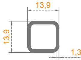
Sistem Kodu: 58-2235 Ağırlık (kg/mt) 0,160
