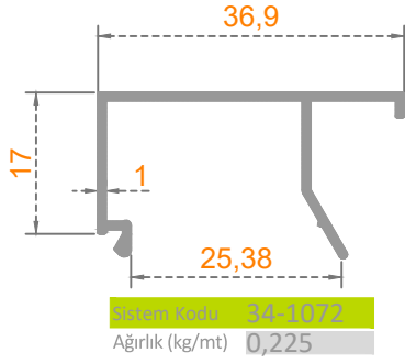
TEK CAM ÇITA
