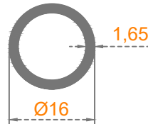
Sistem Kodu: 22-208 Ağırlık (kg/mt) 0,210
