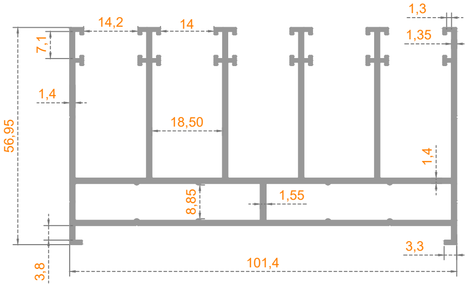
Sistem Kodu: 41-2758 Ağırlık (kg/mt) 2,030
