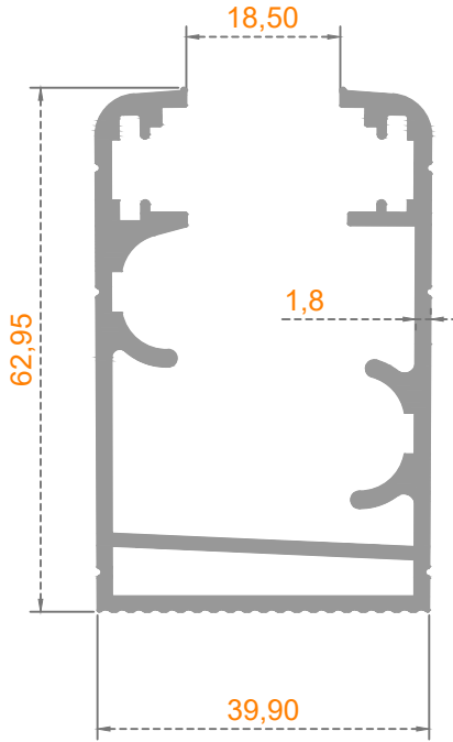
Sistem Kodu: 41-2342 Ağırlık (kg/mt) 1,345
