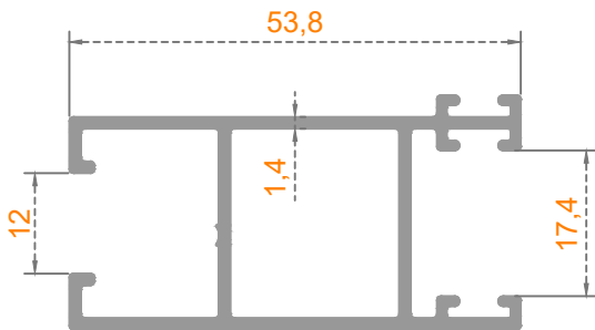
Sistem Kodu: 54-4750 Ağırlık (kg/mt) 0,715
