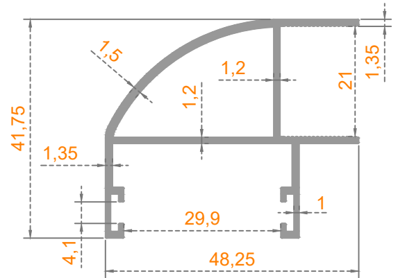
Sistem Kodu: 41-2789 Ağırlık (kg/mt) 0,615
