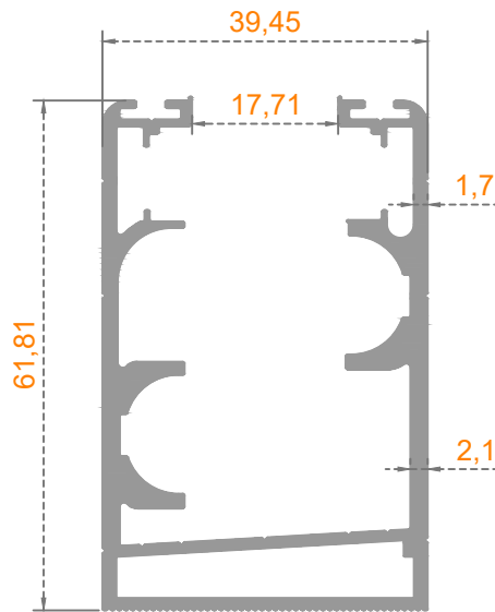
Sistem Kodu: 41-2837 Ağırlık (kg/mt) 1,295
