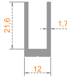
DAR - U -
