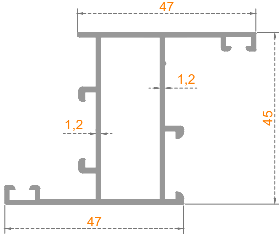
45 'LİK DAR KANAT
