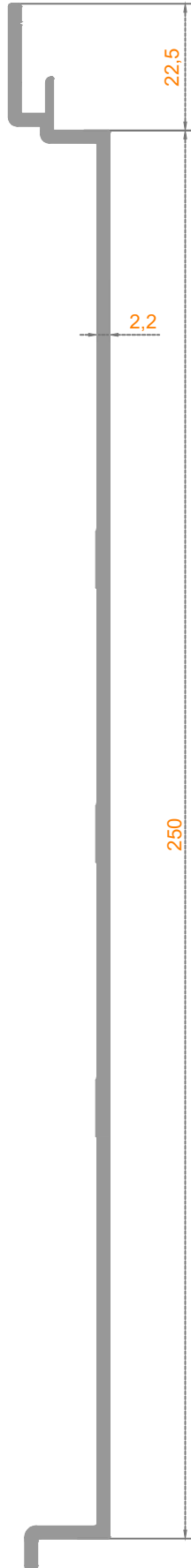
Sistem Kodu: 50-1645 Ağırlık (kg/mt) 1,860
