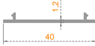
Sistem Kodu: 50-1624 Ağırlık (kg/mt) 0,150
