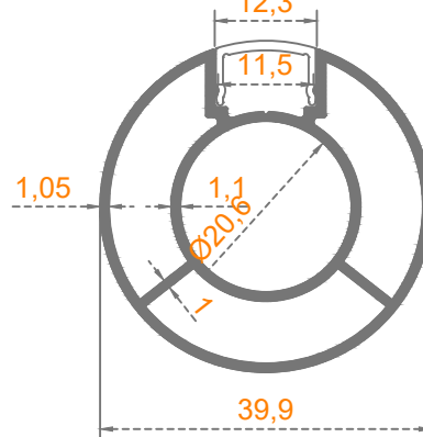
Ø 40'LIK DİKME
