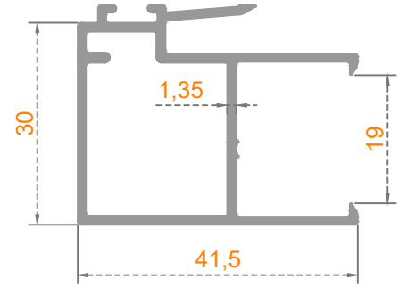
Sistem Kodu: 54-4737 Ağırlık (kg/mt) 0,582
