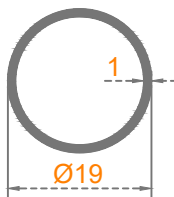
Sistem Kodu: 22-257 Ağırlık (kg/mt) 0,155
