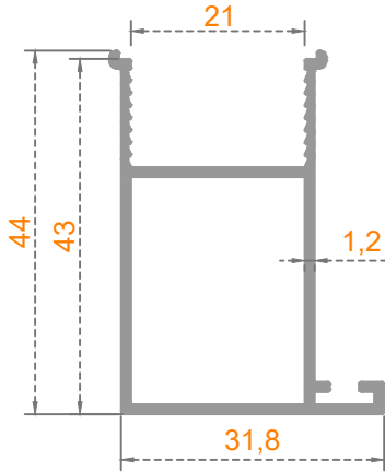
Sistem Kodu: 41-2871 Ağırlık (kg/mt) 0,465
