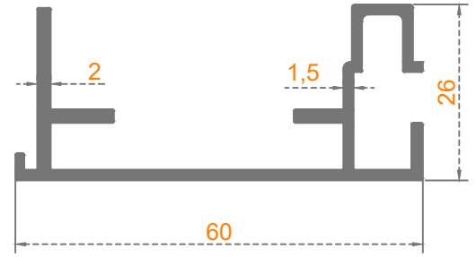
Sistem Kodu: 56-1509 Ağırlık (kg/mt) 0,695
