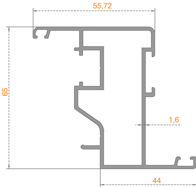
Sistem Kodu: 55-2123 Ağırlık (kg/mt) 1,245
