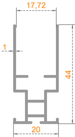
Sistem Kodu: 40-1317 Ağırlık (kg/mt) 0,385
