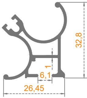
KÖŞE DİKME
