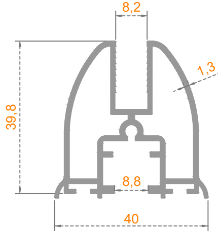
Sistem Kodu: 41-2719 Ağırlık (kg/mt) 0,810
