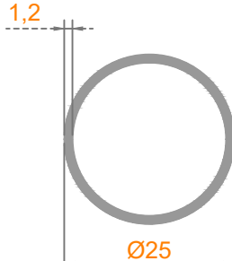
Sistem Kodu: 22-262 Ağırlık (kg/mt) 0,245
