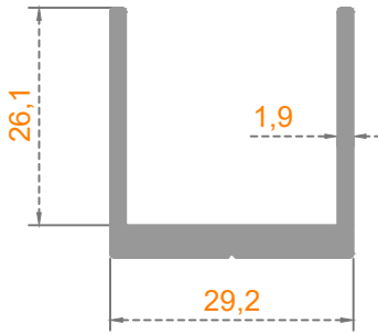
SİSTEM - U -
