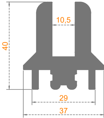
Sistem Kodu: 58-2232 Ağırlık (kg/mt) 1,920
