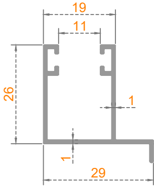
Sistem Kodu: 38-2300 Ağırlık (kg/mt) 0,275
