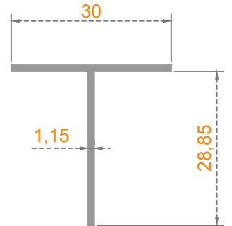
Sistem Kodu: 26-401 Ağırlık (kg/mt) 0,185
