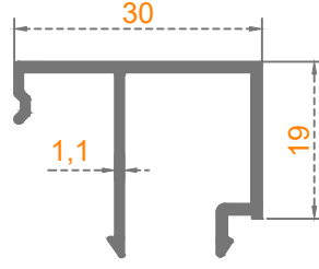
BİM ÇITA
