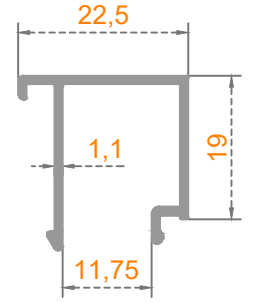
20 MM ISICAM ÇITA
