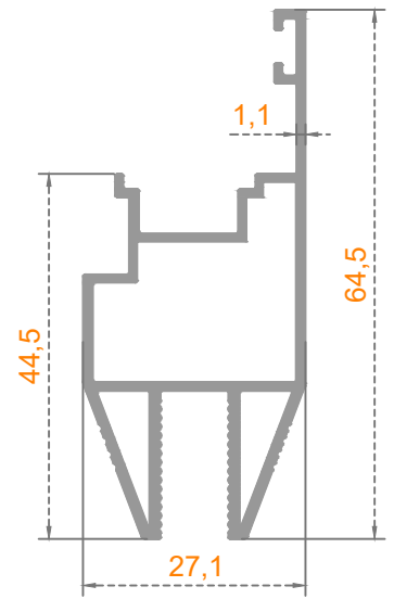
Sistem Kodu: 41-2905 Ağırlık (kg/mt) 0,665
