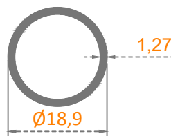
Sistem Kodu: 22-210 Ağırlık (kg/mt) 0,192
