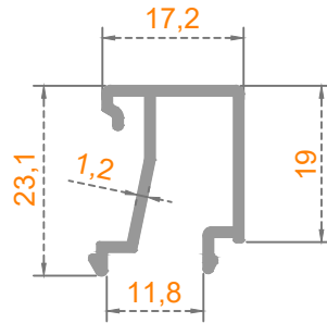
26 MM ÇITA
