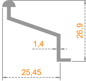
SİNEKLİK RAY
