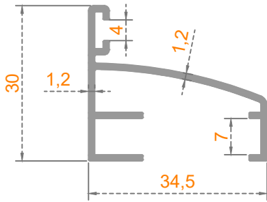
Sistem Kodu: 41-2701 Ağırlık (kg/mt) 0,346
