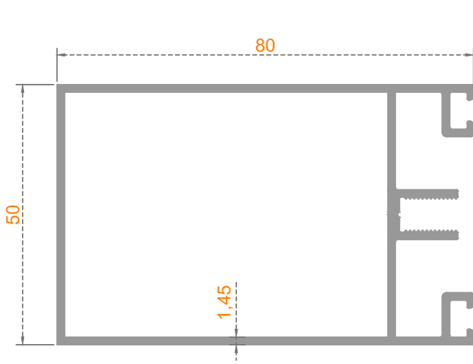
Sistem Kodu: 50-1616 Ağırlık (kg/mt) 1,240
