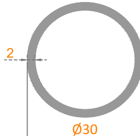
Sistem Kodu: 22-200 Ağırlık (kg/mt) 0,480
