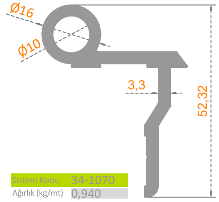
ALDOKS DÜZ KANAT MENTEŞE
