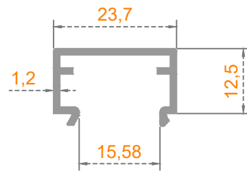
ÜST / YAN RAY
