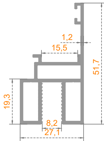
Sistem Kodu: 41-2932 Ağırlık (kg/mt) 0,643
