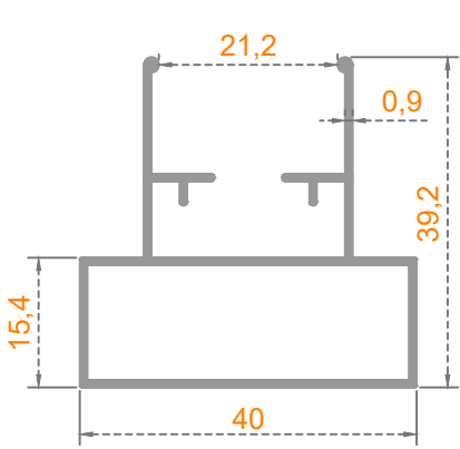
Sistem Kodu: 40-1312-0 Ağırlık (kg/mt) 0,435
