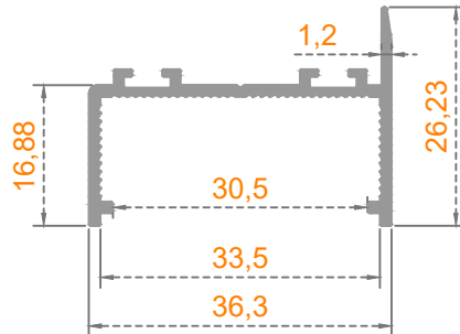
Sistem Kodu: 41-2780 Ağırlık (kg/mt) 0,300
