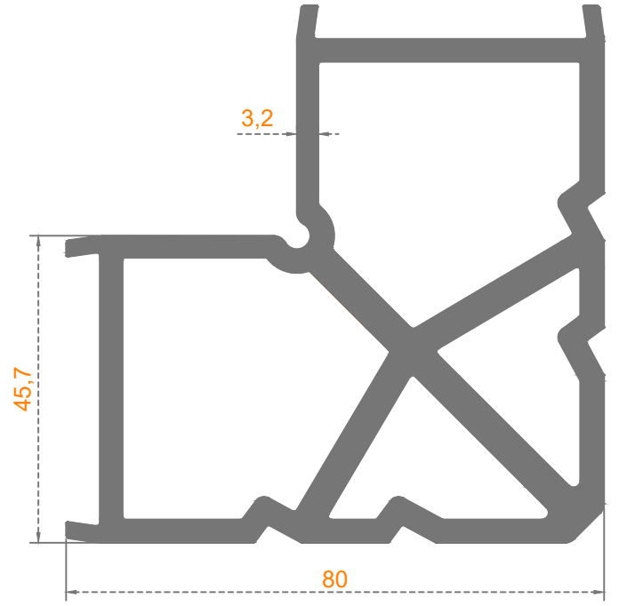
Sistem Kodu: 70-3056 Ağırlık (kg/mt) 4,225
