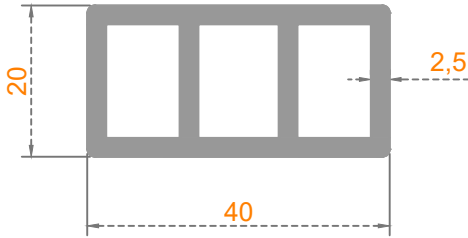
Sistem Kodu: 20-125 Ağırlık (kg/mt) 0,950
