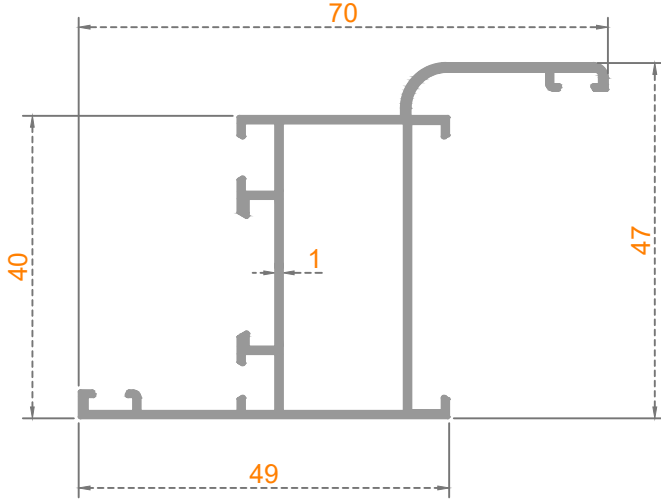
Sistem Kodu: 53-4502 Ağırlık (kg/mt) 0,628
