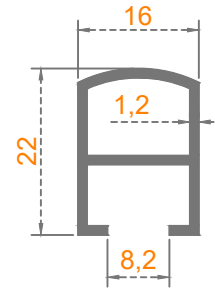
Sistem Kodu: 58-2249 Ağırlık (kg/mt) 0,240
