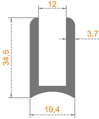
Sistem Kodu: 58-2239 Ağırlık (kg/mt) 0,750
