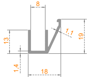
Sistem Kodu: 41-2761 Ağırlık (kg/mt) 0,190
