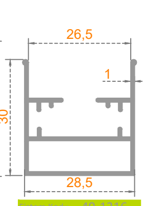
Sistem Kodu: 40-1316 Ağırlık (kg/mt) 0,390
