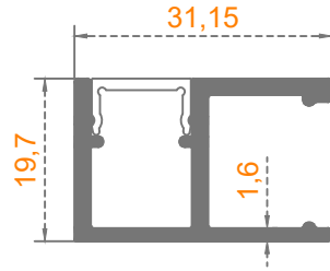
Sistem Kodu: 58-2252 Ağırlık (kg/mt) 0,445
