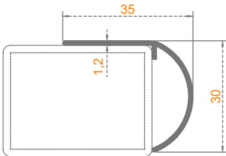
Sistem Kodu: 56-1507 Ağırlık (kg/mt) 0,215
