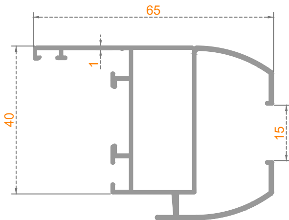
Sistem Kodu: 53-4508 Ağırlık (kg/mt) 0,703
