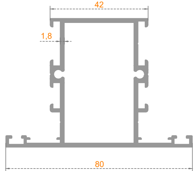
ORTA KAYIT
