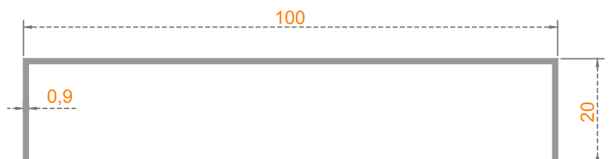
Sistem Kodu: 20-156 Ağırlık (kg/mt) 0,580
