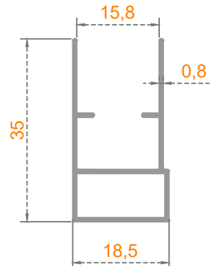
Sistem Kodu: 40-1323 Ağırlık (kg/mt) 0,240
