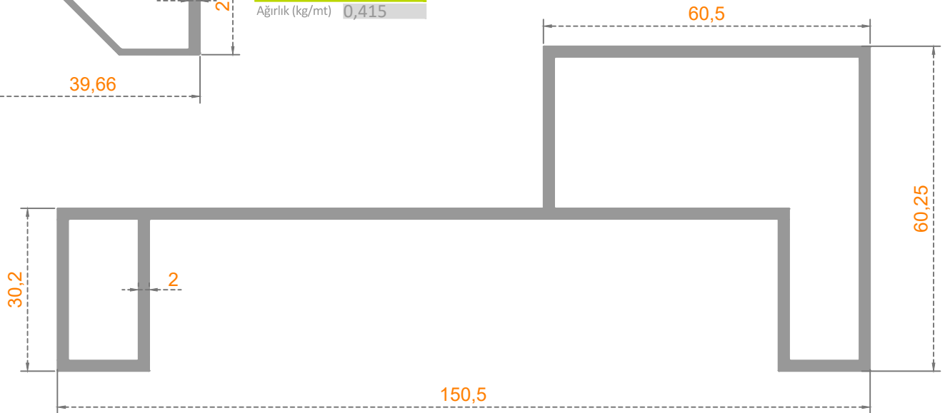
Sistem Kodu: 54-4766 Ağırlık (kg/mt) 2,130
