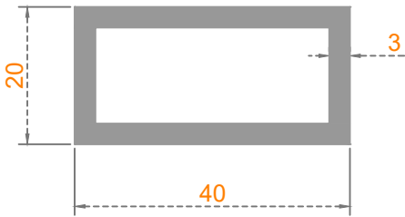
Sistem Kodu: 20-123 Ağırlık (kg/mt) 0,880
