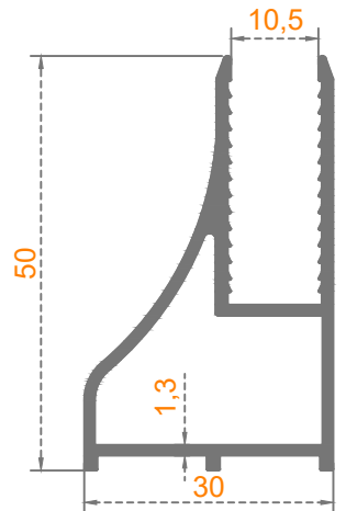
Sistem Kodu: 58-2365 Ağırlık (kg/mt) 0,620
