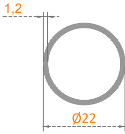
Sistem Kodu: 22-227 Ağırlık (kg/mt) 0,215
