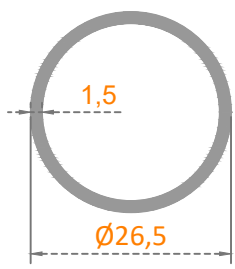
Sistem Kodu: 22-217 Ağırlık (kg/mt) 0,330
