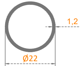
Sistem Kodu: 22-227 Ağırlık (kg/mt) 0,215
