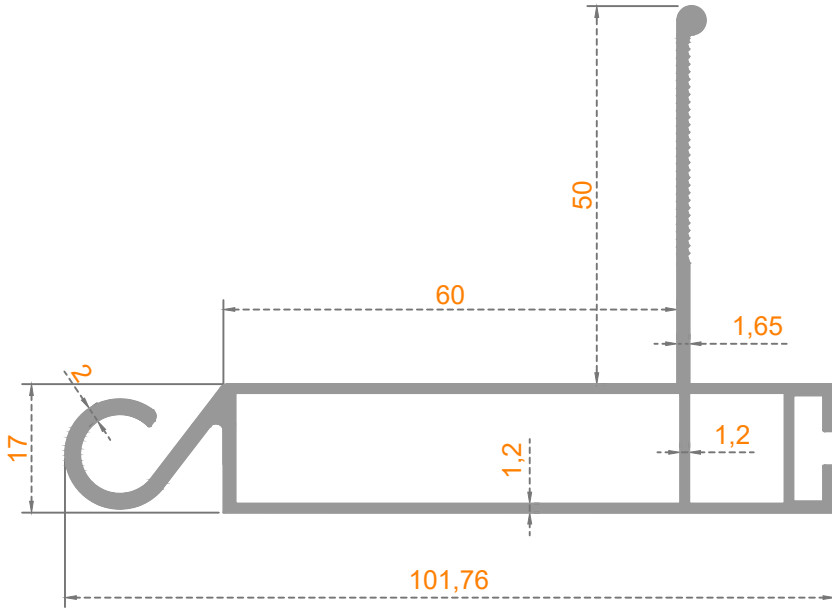
Sistem Kodu: 38-1226 Ağırlık (kg/mt) 1,200
