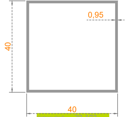
Sistem Kodu: 20-103 Ağırlık (kg/mt) 0,410
