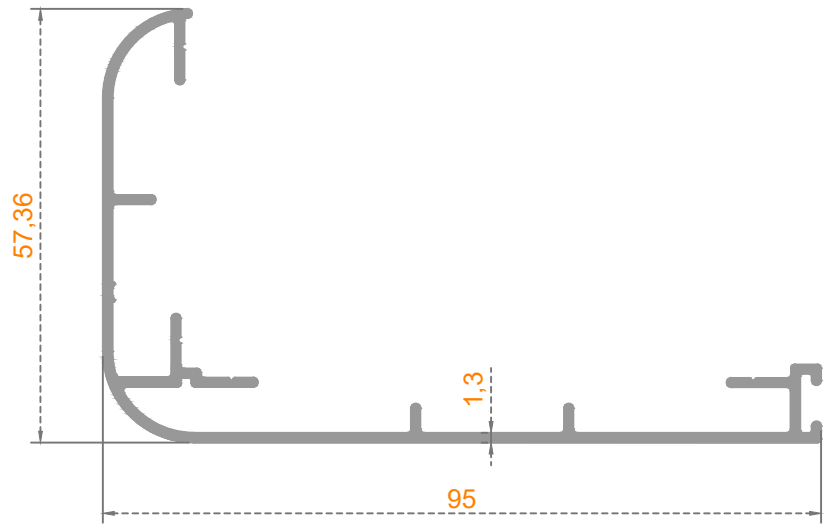
Sistem Kodu: 54-4747 Ağırlık (kg/mt) 0,785
