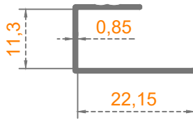
ASMA TAVAN -U-
