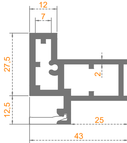
Sistem Kodu: 57-2525 Ağırlık (kg/mt) 1,100
