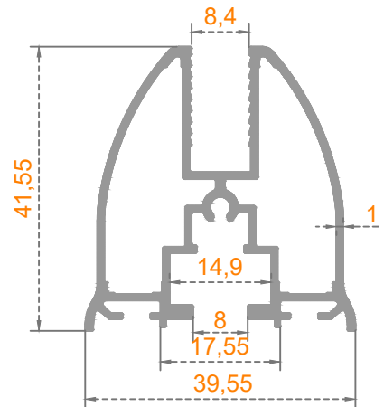
Sistem Kodu: 41-2815 Ağırlık (kg/mt) 0,685
