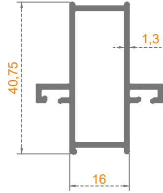
KİLİT PROFİLİ
