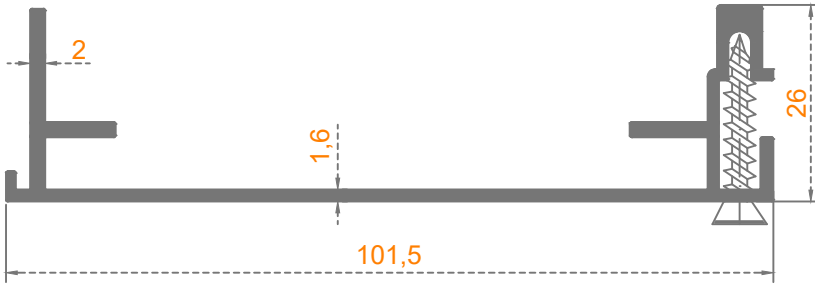
Sistem Kodu: 56-1504 Ağırlık (kg/mt) 0,900
