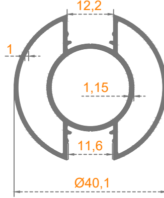
Ø 40'LIK DİKME
