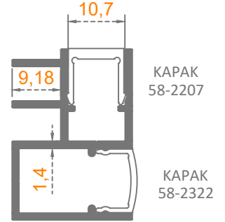
Sistem Kodu: 58-2207 Ağırlık (kg/mt) 0,420
