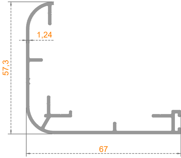
Sistem Kodu: 54-4745 Ağırlık (kg/mt) 0,650
