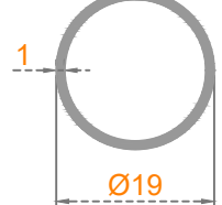
Sistem Kodu: 22-257 Ağırlık (kg/mt) 0,155
