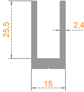
DAR - U -
