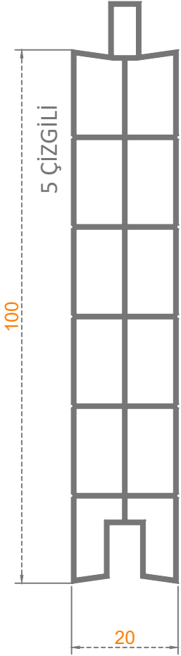
ÇİFT ODACIKLI 10'LUK KAPI LAMBRI
