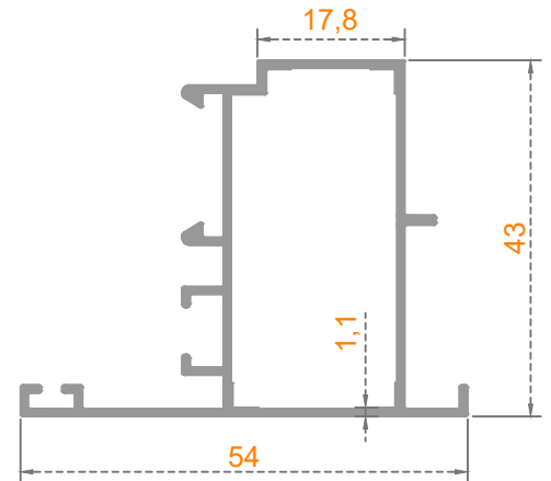
Sistem Kodu: 53-4552 Ağırlık (kg/mt) 0,540
