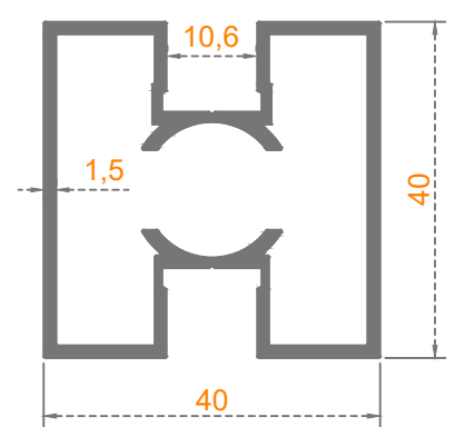
Sistem Kodu: 58-2206 Ağırlık (kg/mt) 0,872
