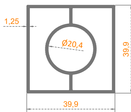
Sistem Kodu: 58-2206 Ağırlık (kg/mt) 0,810
