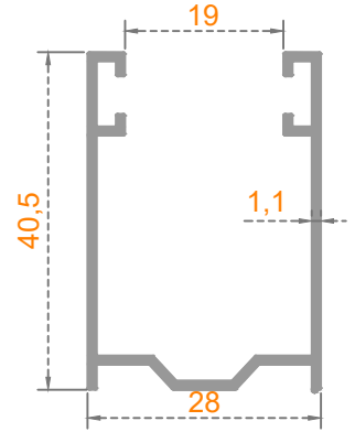
Sistem Kodu: 53-4521 Ağırlık (kg/mt) 0,390
