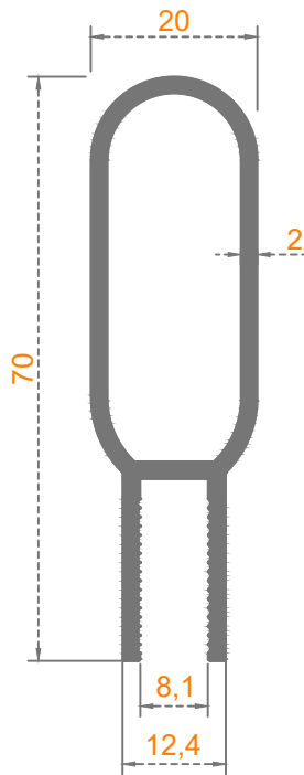
Sistem Kodu: 80-5109 Ağırlık (kg/mt) 0,870
