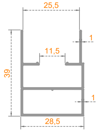
Sistem Kodu: 40-1325 Ağırlık (kg/mt) 0,400
