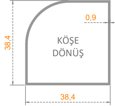
Sistem Kodu: 48-4229 Ağırlık (kg/mt) 0,350
