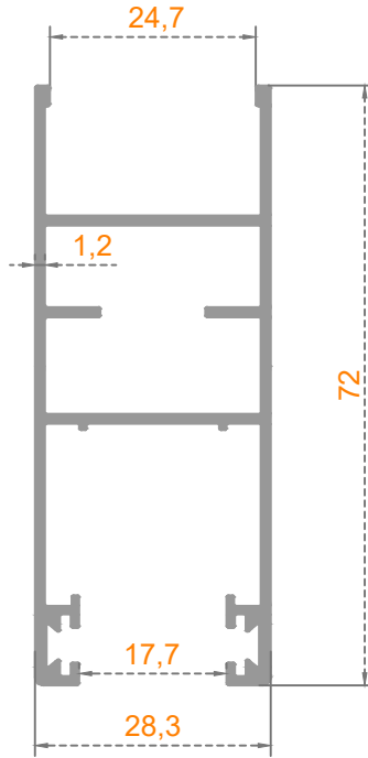
Sistem Kodu: 53-4580 Ağırlık (kg/mt) 0,800
