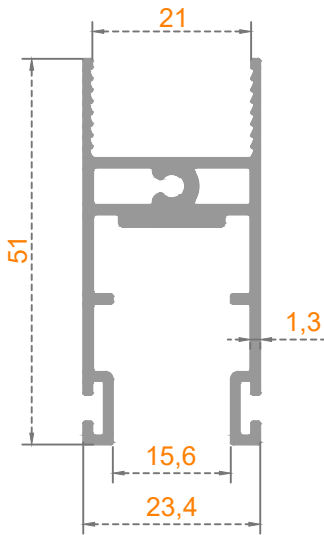
Sistem Kodu: 41-2874 Ağırlık (kg/mt) 0,665
