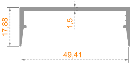
Sistem Kodu: 54-4795 Ağırlık (kg/mt) 0,337
