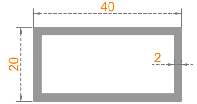
Sistem Kodu: 20-152 Ağırlık (kg/mt) 0,610
