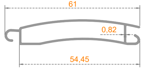
Sistem Kodu: 38-1253 Ağırlık (kg/mt) 0,320
