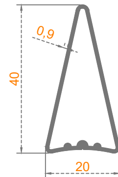
ASMA TAVAN BAĞLANTI PROFİLİ
