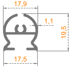
ÖN FİTİLLİ DİKME
