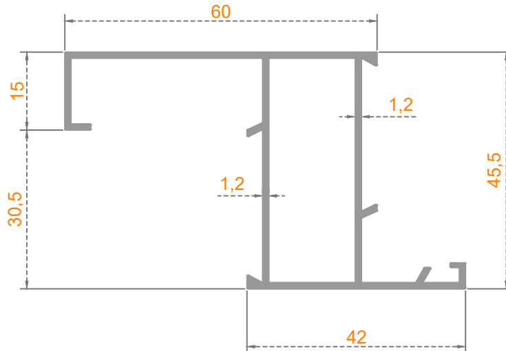
Sistem Kodu: 32-1027 Ağırlık (kg/mt) 0,735
