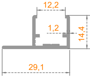
Sistem Kodu: 54-4815 Ağırlık (kg/mt) 0,210
