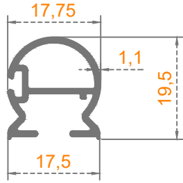
YAN FİTİLLİ DİKME
