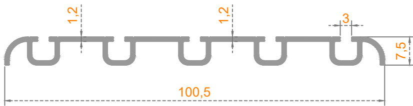
Profil Kodu: 41-2376 Ağırlık (kg/mt) 0,590
