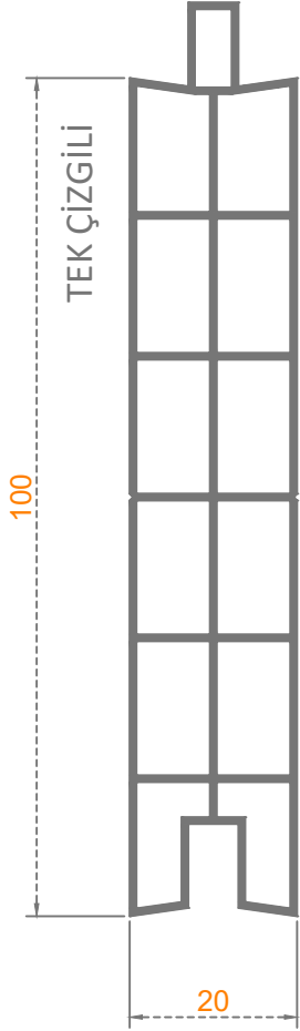
TEK ÇİZGİLİ ÇİFT ODACIKLI 10'LUK KAPI LAMBRI
