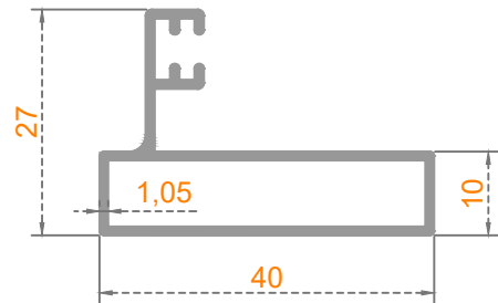
Sistem Kodu: 41-2354 Ağırlık (kg/mt) 0,386
