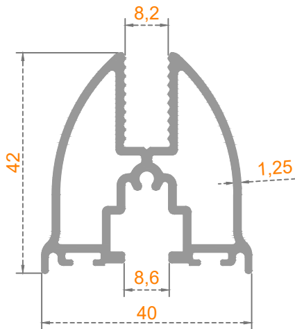
Sistem Kodu: 41-2397 Ağırlık (kg/mt) 0,880
