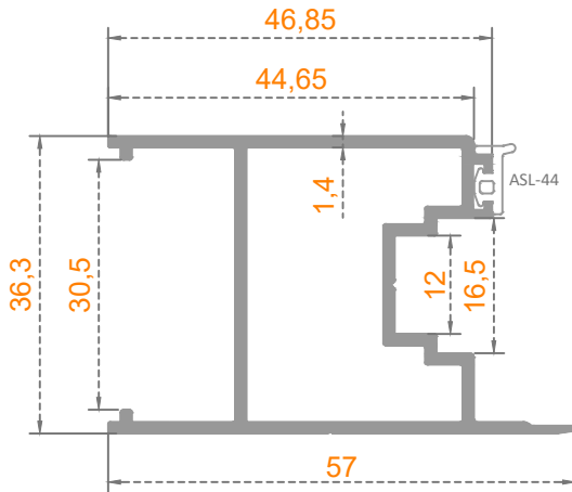
Sistem Kodu: 41-2836 Ağırlık (kg/mt) 0,732
