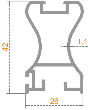
SÜRME DOLAP
