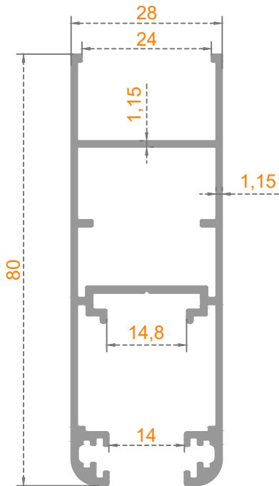
Sistem Kodu: 49-4470 Ağırlık (kg/mt) 0,895
