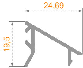
Sistem Kodu: 54-4739 Ağırlık (kg/mt) 0,195
