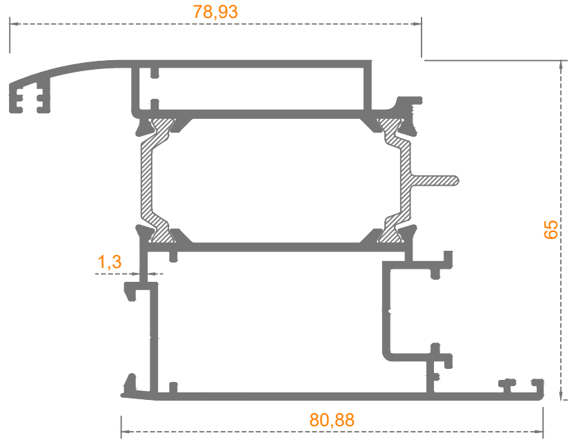
Sistem Kodu: 70-3091 Ağırlık (kg/mt) 1,850
