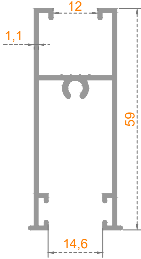
Sistem Kodu: 54-4770 Ağırlık (kg/mt) 0,540
