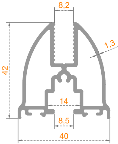
Sistem Kodu: 41-2343 Ağırlık (kg/mt) 0,850
