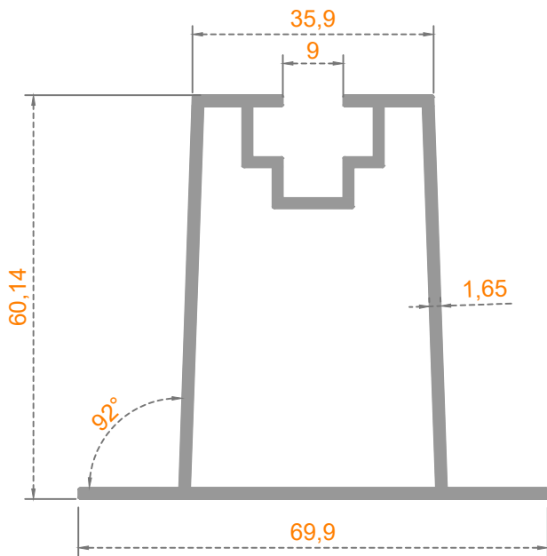
Sistem Kodu 30-524 Ağırlık (kg/mt) 0,900
