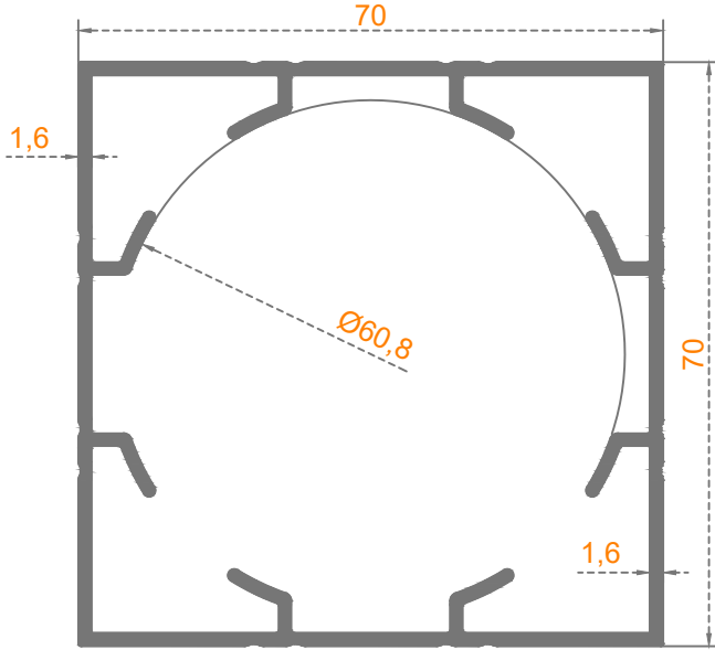
Sistem Kodu: 58-2313 Ağırlık (kg/mt) 1,545
