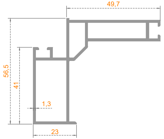
Sistem Kodu: 50-1617 Ağırlık (kg/mt) 0,955
