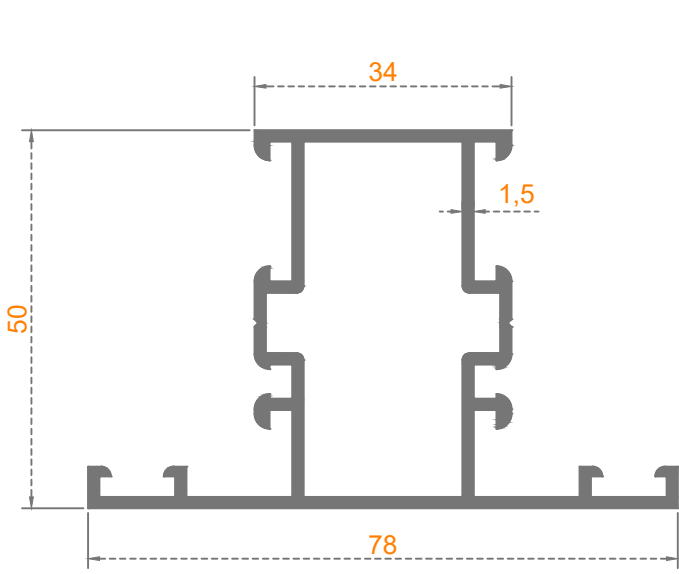
ORTA KAYIT
