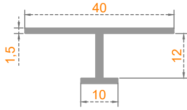
Sistem Kodu: 26-411 Ağırlık (kg/mt) 0,270
