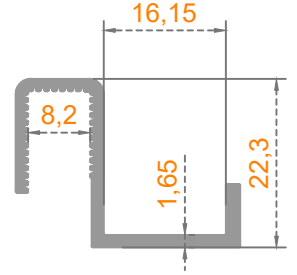
Sistem Kodu: 80-5258 Ağırlık (kg/mt) 0,303
