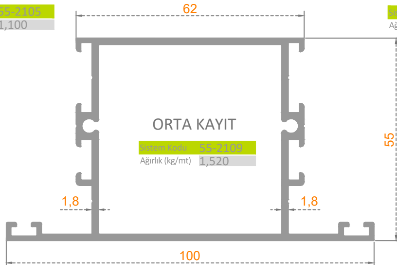
ORTA KAYIT
