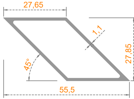
Sistem Kodu: 20-159 Ağırlık (kg/mt) 0,390
