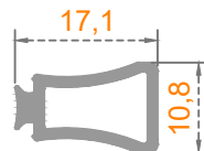
Sistem Kodu: 41-2877 Ağırlık (kg/mt) 0,165
