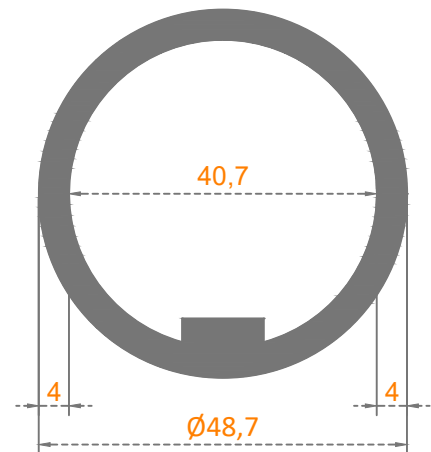
Ø 40'LIK DİKME FLANŞI
