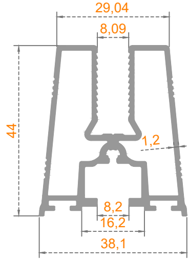
Sistem Kodu: 41-2929 Ağırlık (kg/mt) 0,854
