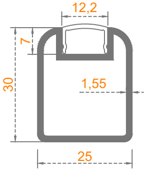
Sistem Kodu: 58-2262 Ağırlık (kg/mt) 0,460
