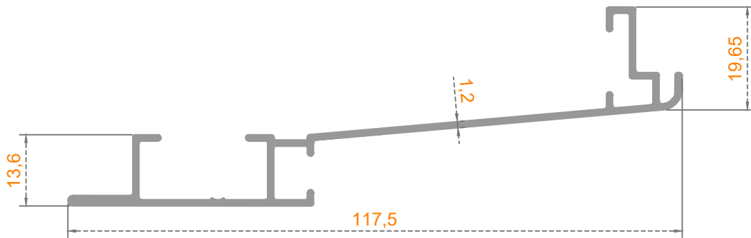
Sistem Kodu: 54-4746 Ağırlık (kg/mt) 0,770
