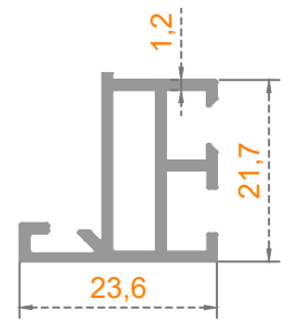
Sistem Kodu: 50-1618 Ağırlık (kg/mt) 0,320
