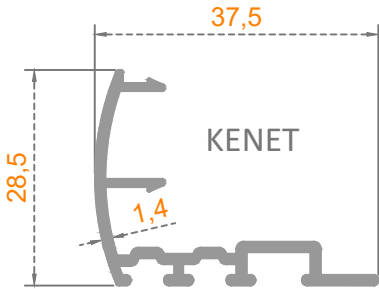
Sistem Kodu: 47-4013 Ağırlık (kg/mt) 0,355
