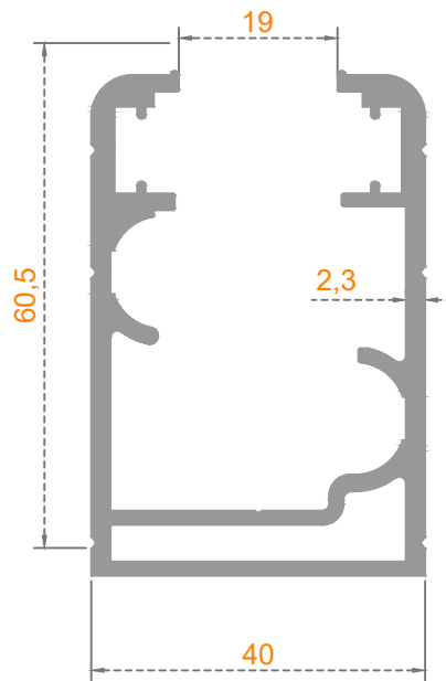
Sistem Kodu 41-2352 Ağırlık (kg/mt) 1,431
