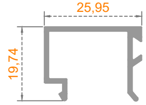
Sistem Kodu: 54-4762 Ağırlık (kg/mt) 0,251
