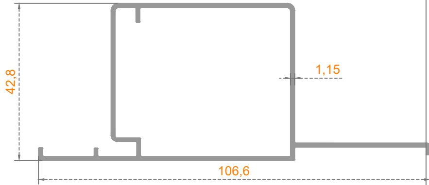
Sistem Kodu: 50-1653 Ağırlık (kg/mt) 0,780
