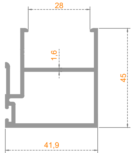
Sistem Kodu: 54-4821 Ağırlık (kg/mt) 0,860
