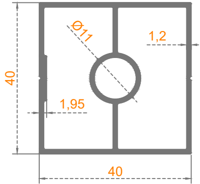
Sistem Kodu: 58-2317 Ağırlık (kg/mt) 0,735
