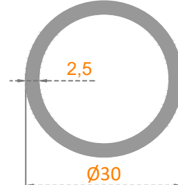
Sistem Kodu: 22-201 Ağırlık (kg/mt) 0,586
