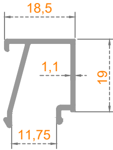
24 MM ÇITA
