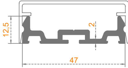
ALT ADAPTÖR
