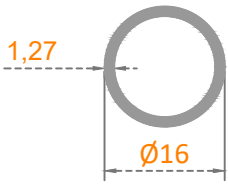
Sistem Kodu: 22-230 Ağırlık (kg/mt) 0,160
