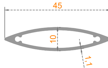
GÜNEŞ KIRICI
