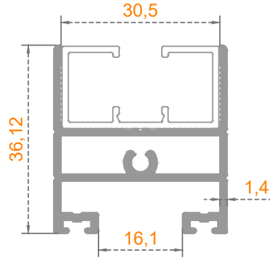
Sistem Kodu: 41-2852 Ağırlık (kg/mt) 0,621
