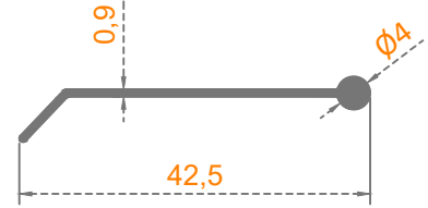
MENFEZ KANAT
