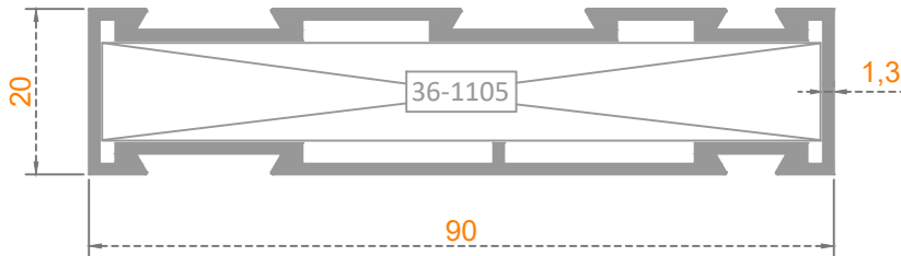
SİNEKLİKLİ KASA
