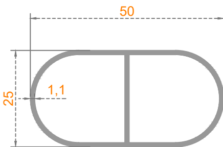
Sistem Kodu: 22-251 Ağırlık (kg/mt) 0,440
