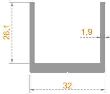
GENİŞ - U -
