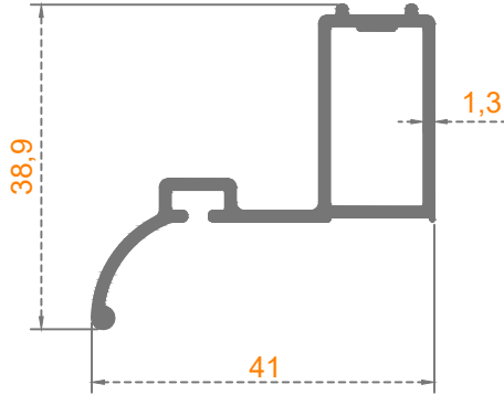
KÜÇÜK BAĞLI DİKME
