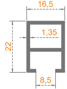
Sistem Kodu: 58-2281 Ağırlık (kg/mt) 0,285
