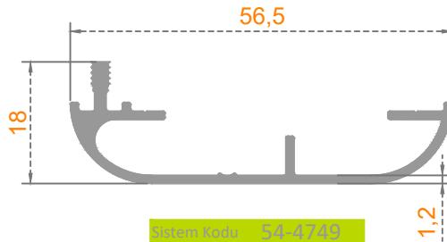
Sistem Kodu: 54-4749 Ağırlık (kg/mt) 0,376
