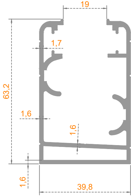
Sistem Kodu 41-2398 Ağırlık (kg/mt) 1,253
