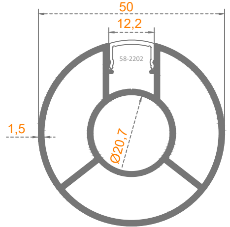
Ø 50'LIK DİKME
