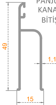
Sistem Kodu: 47-4024 Ağırlık (kg/mt) 0,300
