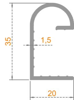
Sistem Kodu: 48-4224 Ağırlık (kg/mt) 0,335
