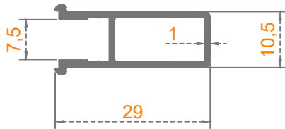
ÇERÇEVE DİKME
