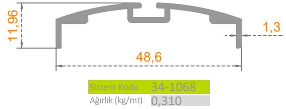
ÇARPMA KAPI DIŞ
