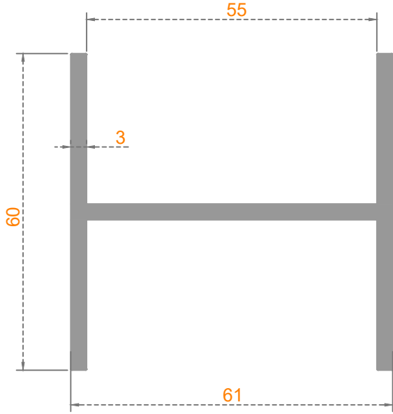
Sistem Kodu: 26-404 Ağırlık (kg/mt) 1,425
