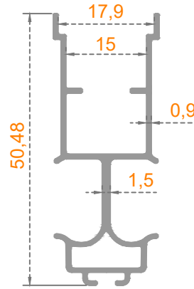
Sistem Kodu: 40-1324 Ağırlık (kg/mt) 0,370
