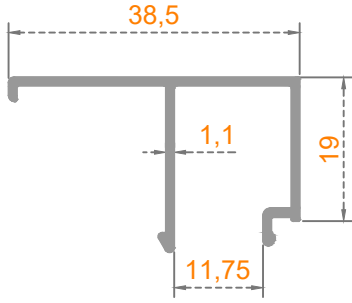
4 MM TEK CAM ÇITA
