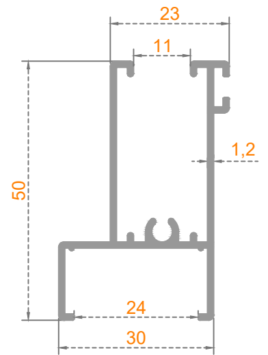
ISICAMLI KANAT ALT / ÜST
