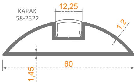
Sistem Kodu: 58-2322 Ağırlık (kg/mt) 0,495
