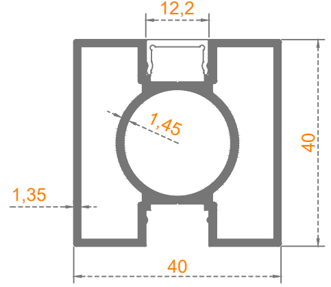
Sistem Kodu: 58-2224 Ağırlık (kg/mt) 0,925
