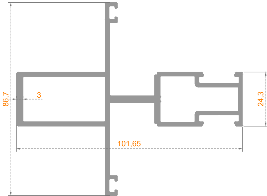
Sistem Kodu: 54-4778 Ağırlık (kg/mt) 1,997
