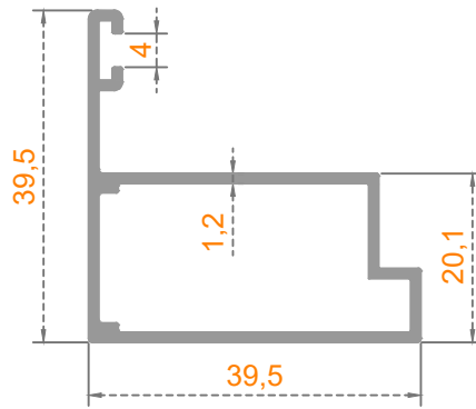
Sistem Kodu: 41-2704 Ağırlık (kg/mt) 0,475
