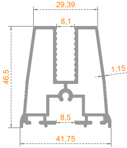
Sistem Kodu: 41-2906 Ağırlık (kg/mt) 0,918
