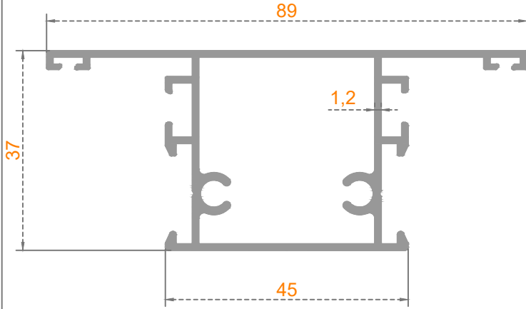
Sistem Kodu: 49-4408 Ağırlık (kg/mt) 0,945
