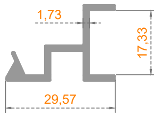
Sistem Kodu: 50-1619 Ağırlık (kg/mt) 0,335
