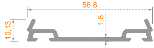
Sistem Kodu: 50-11006 Ağırlık (kg/mt) 0,405
