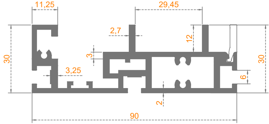
Sistem Kodu: 57-2524 Ağırlık (kg/mt) 1,970
