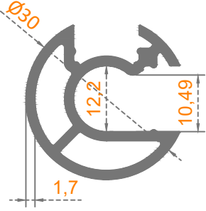
Ø 30'LUK DİKME
