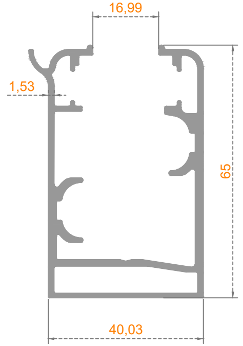
Sistem Kodu: 41-2829 Ağırlık (kg/mt) 1,268
