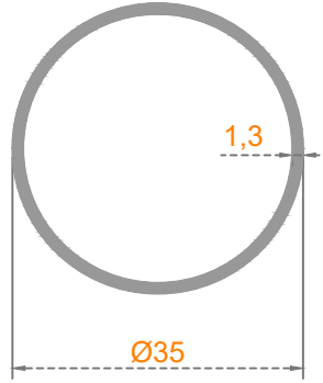
Sistem Kodu: 22-255 Ağırlık (kg/mt) 0,375
