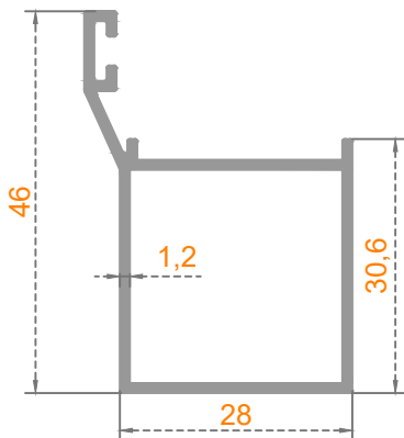
Sistem Kodu: 41-2876 Ağırlık (kg/mt) 0,460
