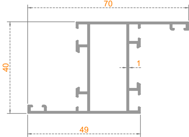
Sistem Kodu: 53-4501 Ağırlık (kg/mt) 0,638
