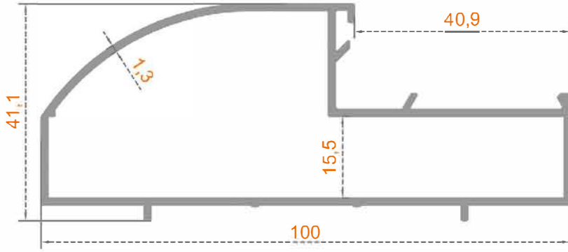
Sistem Kodu: 38-1272 Ağırlık (kg/mt) 1,010
