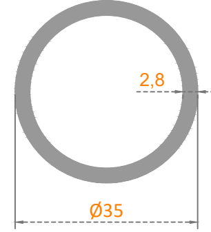
Sistem Kodu: 22-206 Ağırlık (kg/mt) 0,770
