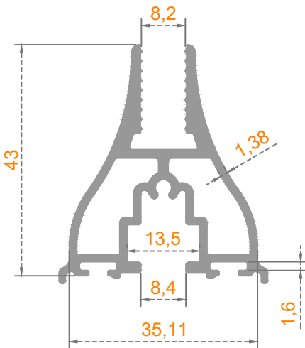
Sistem Kodu: 41-2724 Ağırlık (kg/mt) 0,880
