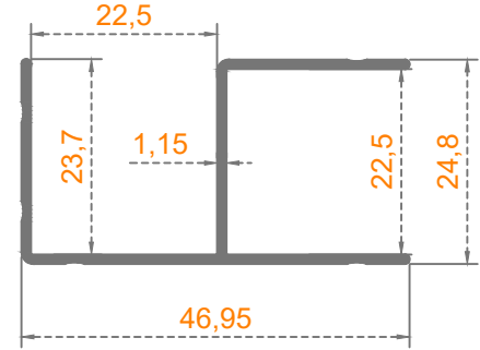
BAĞLI DİKME
