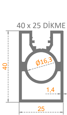
Sistem Kodu: 58-2243 Ağırlık (kg/mt) 0,790
