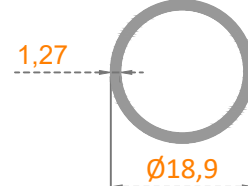
Sistem Kodu: 22-231 Ağırlık (kg/mt) 0,192
