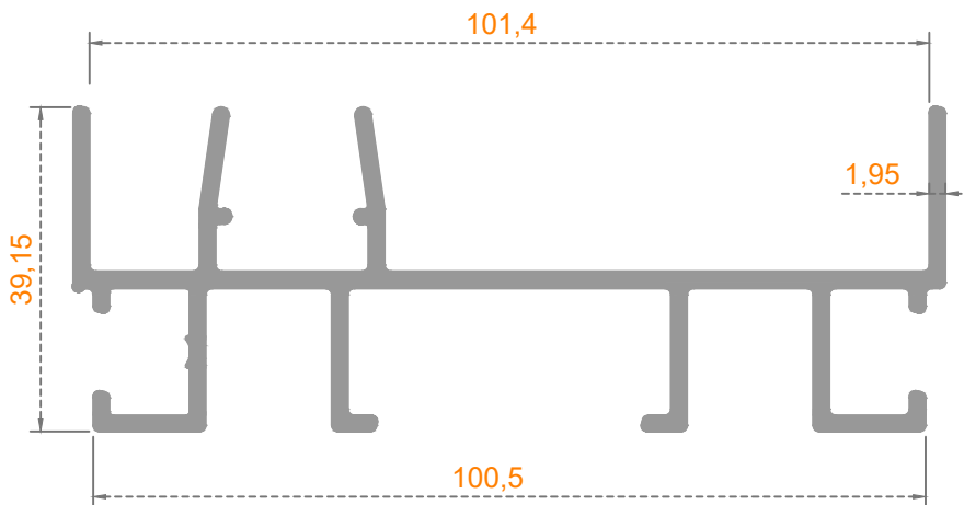
Sistem Kodu: 54-4731 Ağırlık (kg/mt) 0,720
