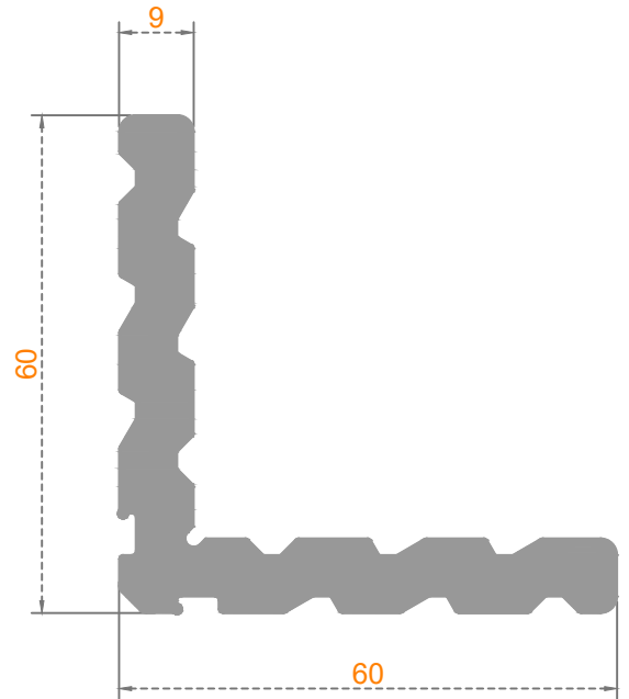
Sistem Kodu: 50-1471 Ağırlık (kg/mt) 2,350
