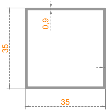
Sistem Kodu: 20-153 Ağırlık (kg/mt) 0,335
