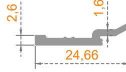
Sistem Kodu: 54-4784 Ağırlık (kg/mt) 0,133
