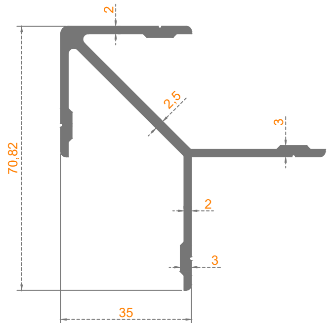
C-60 ÇAVUŞ
