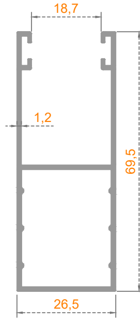
Sistem Kodu: 38-1224 Ağırlık (kg/mt) 0,685
