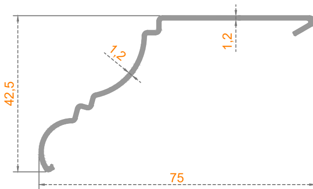
Sistem Kodu: 48-4223 Ağırlık (kg/mt) 0,365
