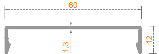
Sistem Kodu: 27-11005 Ağırlık (kg/mt) 0,305
