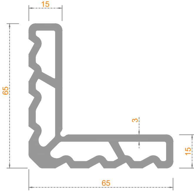
S.ÇERÇEVE TAKOZU
