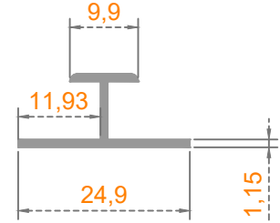
Sistem Kodu: 39-1288 Ağırlık (kg/mt) 0,132
