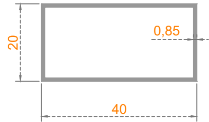
Sistem Kodu: 20-101 Ağırlık (kg/mt) 0,275
