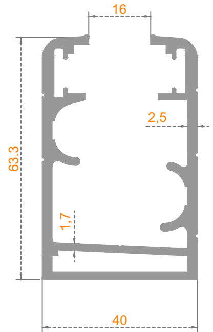
Sistem Kodu 41-2450 Ağırlık (kg/mt) 1,625
