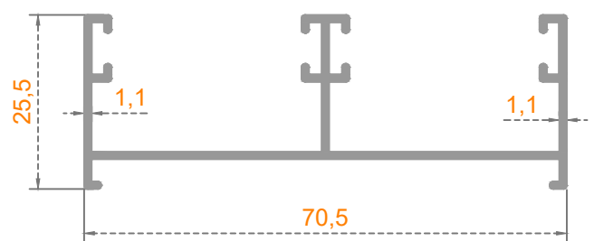
KASA ÜST
