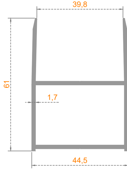
Sistem Kodu: 41-1306 Ağırlık (kg/mt) 0,935
