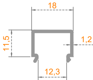
ÜST / YAN RAY
