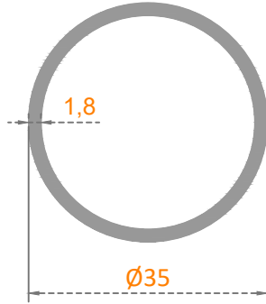
Sistem Kodu: 22-234 Ağırlık (kg/mt) 0,510
