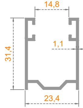
Sistem Kodu: 53-4520 Ağırlık (kg/mt) 0,320
