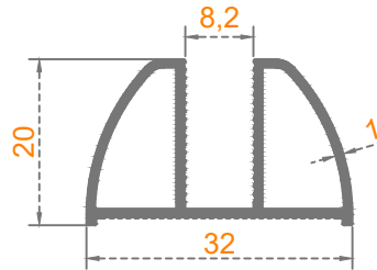
Sistem Kodu: 58-2316 Ağırlık (kg/mt) 0,320
