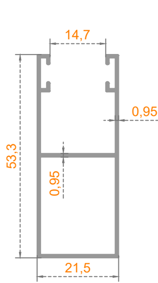
Sistem Kodu: 38-1218 Ağırlık (kg/mt) 0,422
