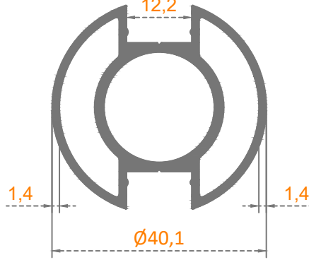
Ø 40'LIK DİKME
