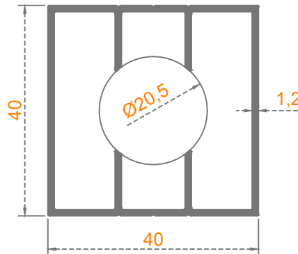
Sistem Kodu: 58-2370 Ağırlık (kg/mt) 0,649
