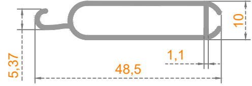
FİTİLLİ ALT PARÇA
