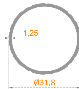
Sistem Kodu: 80-5026 Ağırlık (kg/mt) 0,315
