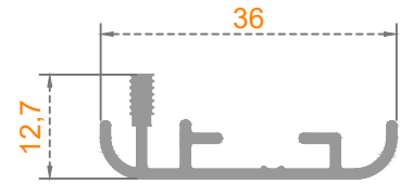
Sistem Kodu: 54-4742 Ağırlık (kg/mt) 0,250
