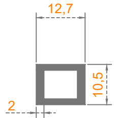
Sistem Kodu: 41-2381 Ağırlık (kg/mt) 0,190
