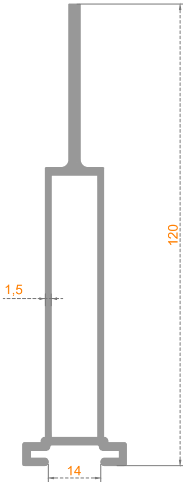
Sistem Kodu: 50-1659 Ağırlık (kg/mt) 1,220
