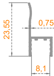
Sistem Kodu: 41-2494 Ağırlık (kg/mt) 0,100
