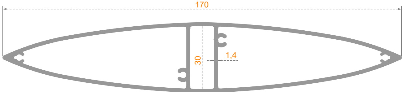
GÜNEŞ KIRICI
