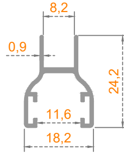
Sistem Kodu: 41-2395 Ağırlık (kg/mt) 0,190
