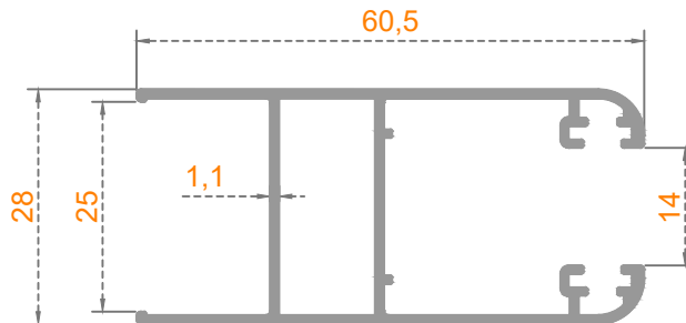
Sistem Kodu: 47-4015 Ağırlık (kg/mt) 0,625
