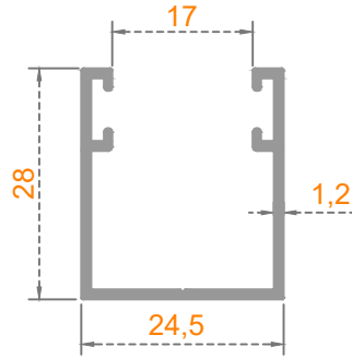
Sistem Kodu: 53-4518 Ağırlık (kg/mt) 0,305
