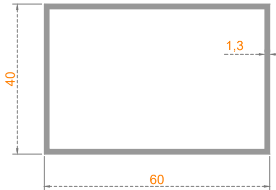
Sistem Kodu: 20-122 Ağırlık (kg/mt) 0,700
