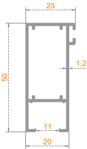
TEK CAMLI KANAT YAN
