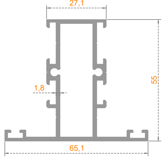
ORTA KAYIT
