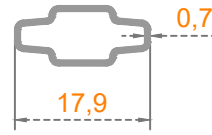
KAROLAJ ÇİTASI
