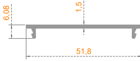
Sistem Kodu: 38-1215 Ağırlık (kg/mt) 0,250
