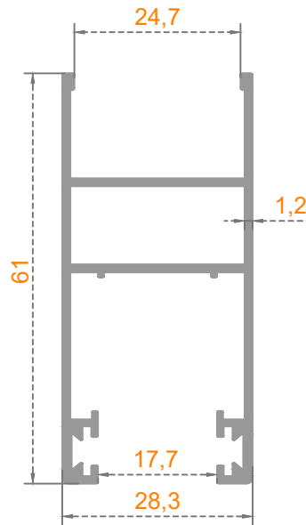
Sistem Kodu: 53-4574 Ağırlık (kg/mt) 0,685
