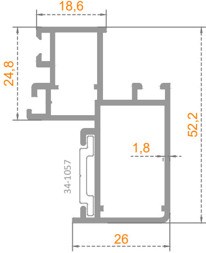
Sistem Kodu: 50-1488 Ağırlık (kg/mt) 0,776
