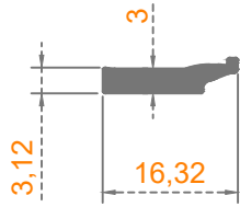
Sistem Kodu: 57-2523 Ağırlık (kg/mt) 0,125
