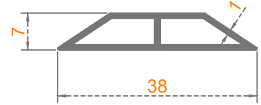
Sistem Kodu: 80-5042 Ağırlık (kg/mt) 0,220
