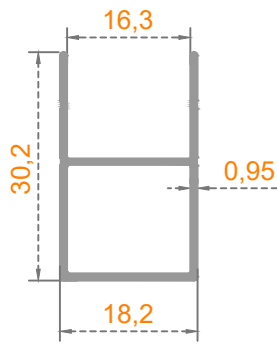
Sistem Kodu: 40-1329 Ağırlık (kg/mt) 0,235
