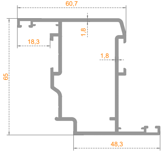
FUGALI KANAT
