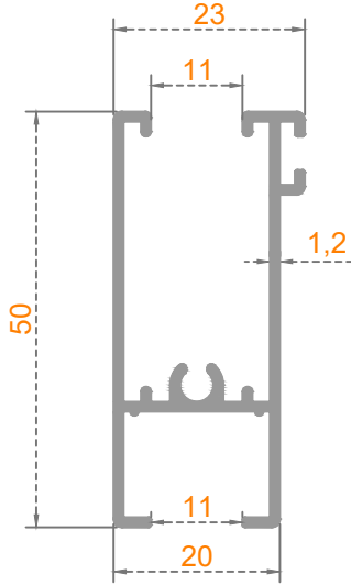
TEK CAMLI KANAT ALT / ÜST
