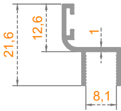
Sistem Kodu: 41-2394 Ağırlık (kg/mt) 0,145
