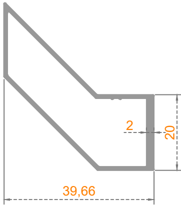
Sistem Kodu: 54-4798 Ağırlık (kg/mt) 0,415
