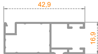
Sistem Kodu: 40-1303 Ağırlık (kg/mt) 0,325
