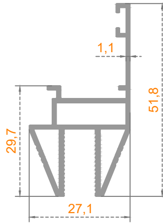
Sistem Kodu: 41-2904 Ağırlık (kg/mt) 0,558
