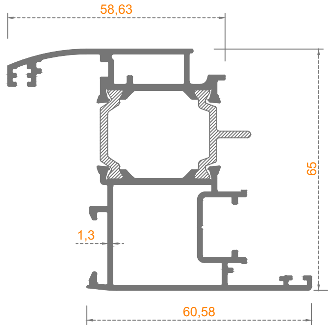
Sistem Kodu: 70-3092 Ağırlık (kg/mt) 1,525
