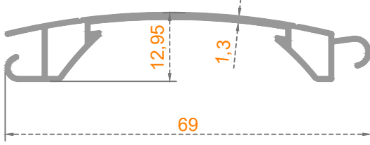
Sistem Kodu: 38-1207 Ağırlık (kg/mt) 0,385
