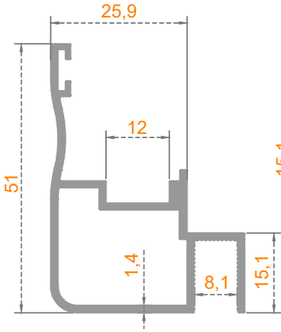
Sistem Kodu: 41-2798 Ağırlık (kg/mt) 0,615
