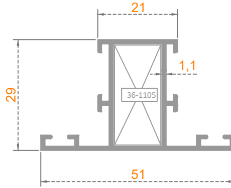
ORTA KAYIT
