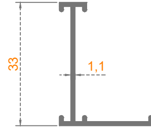
TAŞIYICI -L-
