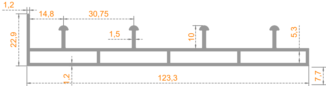
Sistem Kodu: 41-2869 Ağırlık (kg/mt) 0,875
