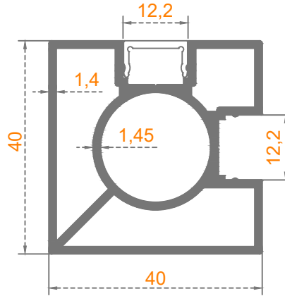
Sistem Kodu: 58-2264 Ağırlık (kg/mt) 1,000
