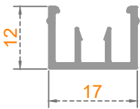
Sistem Kodu: 50-1626 Ağırlık (kg/mt) 0,168
