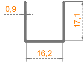
ASMA TAVAN -U-
