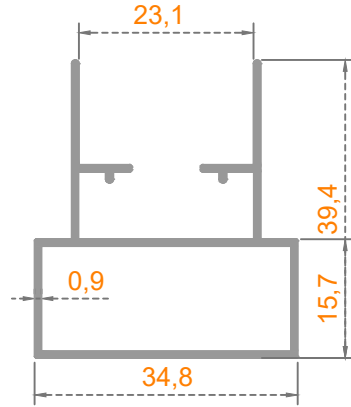
Sistem Kodu: 40-1320 Ağırlık (kg/mt) 0,400
