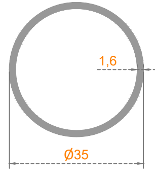
Sistem Kodu: 58-2332 Ağırlık (kg/mt) 0,460
