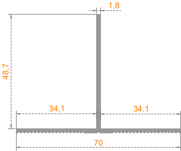
Sistem Kodu: 50-1640 Ağırlık (kg/mt) 0,540
