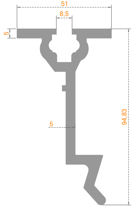
Sistem Kodu 30-529 Ağırlık (kg/mt) 2,370
