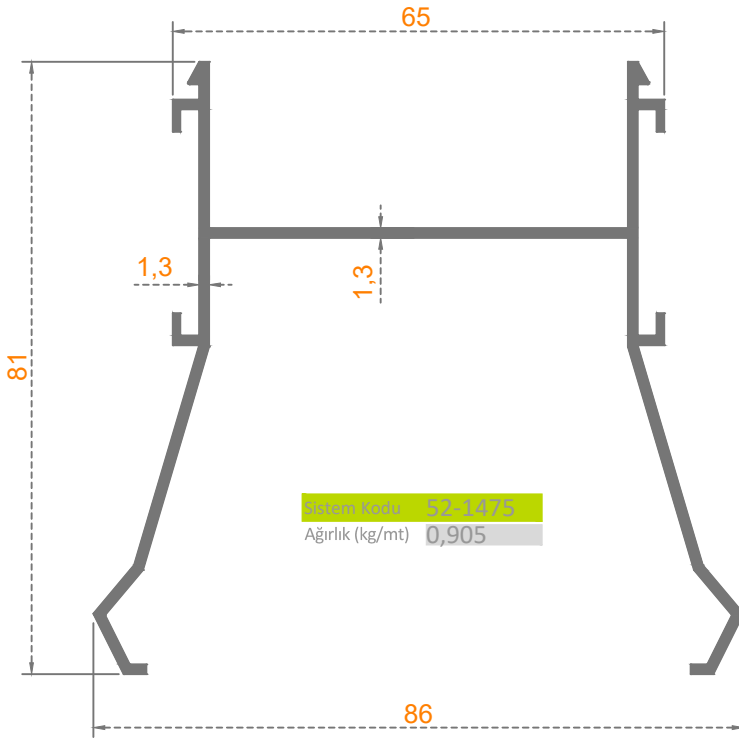
LAMBA -H- PROFİLİ
