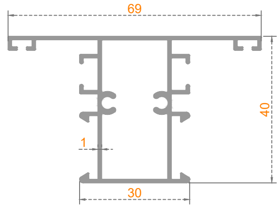
Sistem Kodu: 53-4553 Ağırlık (kg/mt) 0,700
