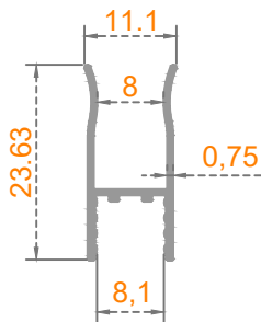
Sistem Kodu: 41-2493 Ağırlık (kg/mt) 0,130
