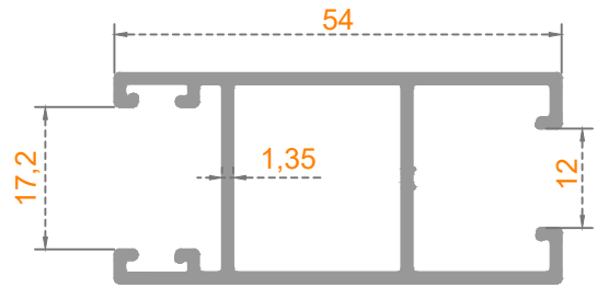
Sistem Kodu: 54-4733 Ağırlık (kg/mt) 0,670
