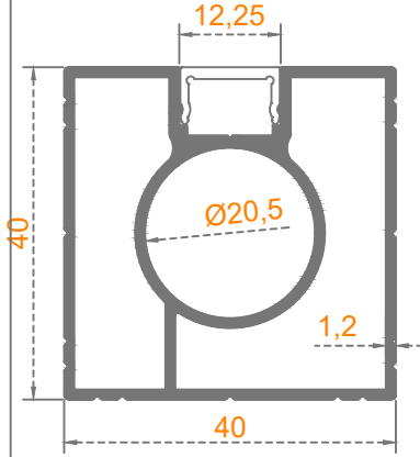
Sistem Kodu: 58-2312 Ağırlık (kg/mt) 0,805
