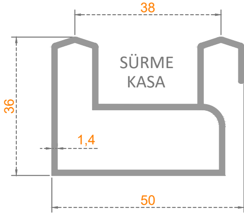
Sistem Kodu: 47-4025 Ağırlık (kg/mt) 0,710
