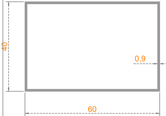
Sistem Kodu: 20-144 Ağırlık (kg/mt) 0,480
