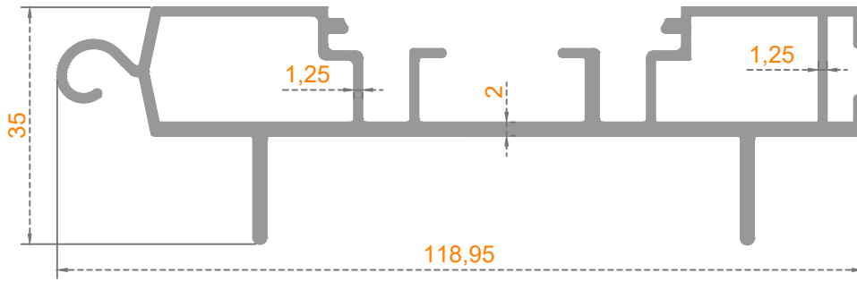
Sistem Kodu: 38-1214 Ağırlık (kg/mt) 1,445
