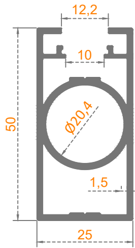
Sistem Kodu: 58-2295 Ağırlık (kg/mt) 0,885
