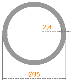
Sistem Kodu: 22-223 Ağırlık (kg/mt) 0,675
