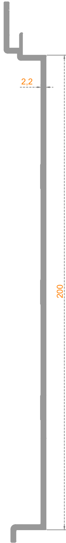
Sistem Kodu: 50-1611 Ağırlık (kg/mt) 1,561
