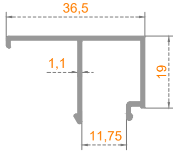
6 ve 8 MM ÇITA
