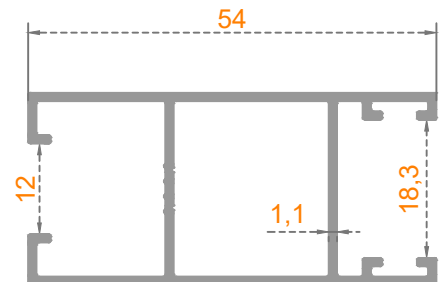
Sistem Kodu: 54-4772 Ağırlık (kg/mt) 0,554
