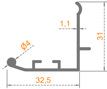
MENFEZ KASA
