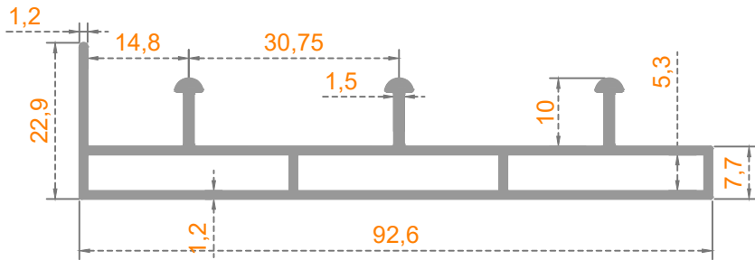
Sistem Kodu: 41-2869 Ağırlık (kg/mt) 0,875
