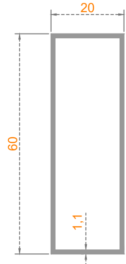
Sistem Kodu: 20-112 Ağırlık (kg/mt) 0,470
