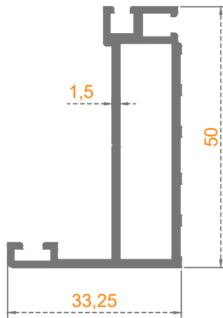
KAPAKLI CEPHE DIŞA AÇILIR KASA
