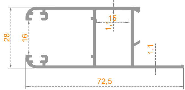
Sistem Kodu: 47-4027 Ağırlık (kg/mt) 0,635
