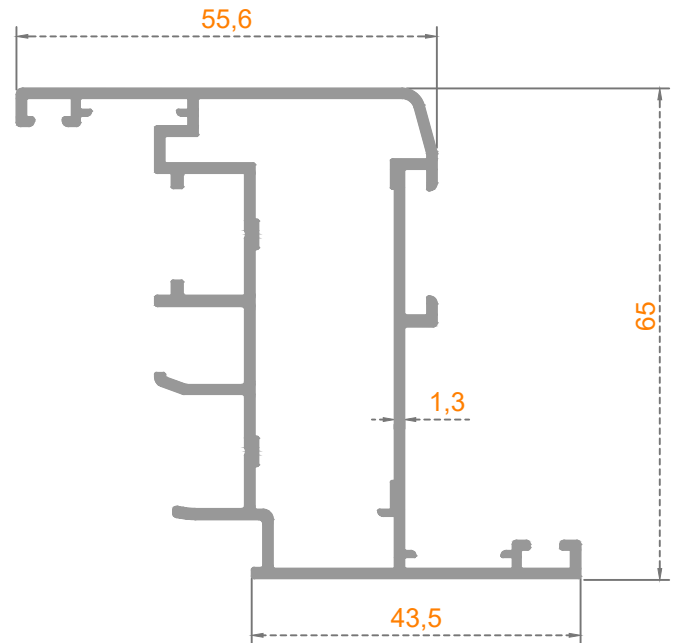
Sistem Kodu: 55-2135 Ağırlık (kg/mt) 1,140
