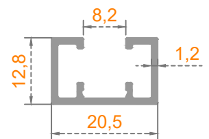
Sistem Kodu: 41-2875 Ağırlık (kg/mt) 0,200
