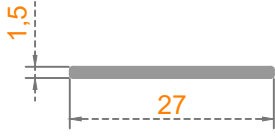
Sistem Kodu: 41-2831 Ağırlık (kg/mt) 0,110
