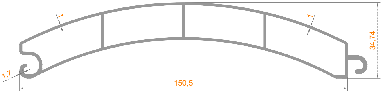
Sistem Kodu: 38-1222 Ağırlık (kg/mt) 1,200
