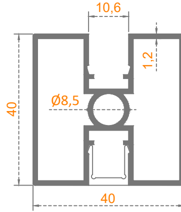
Sistem Kodu: 58-2255 Ağırlık (kg/mt) 0,775
