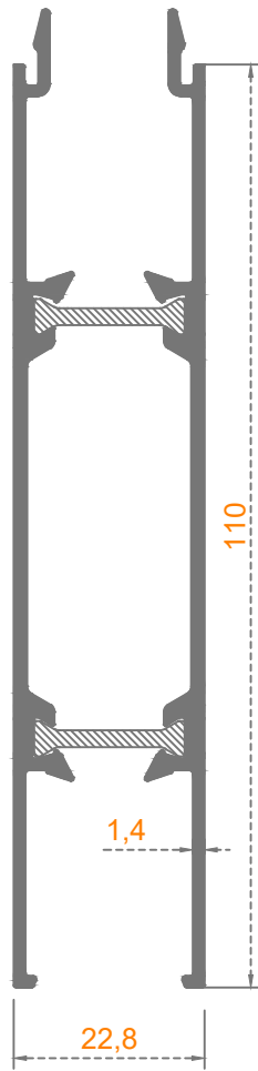
Sistem Kodu: 70-3093 Ağırlık (kg/mt) 1,365
