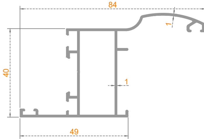
Sistem Kodu: 53-4516 Ağırlık (kg/mt) 0,655
