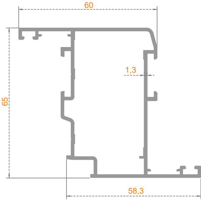
FUGALI KANAT
