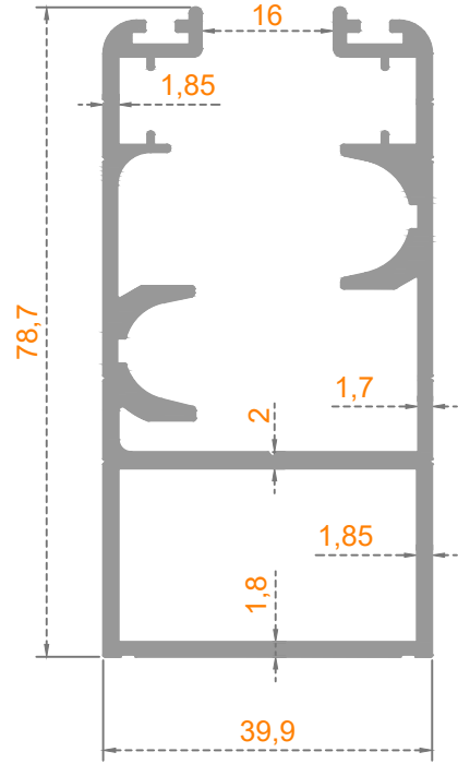
Sistem Kodu 41-2765 Ağırlık (kg/mt) 1,615
