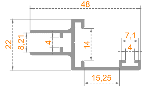
Sistem Kodu: 41-2842 Ağırlık (kg/mt) 0,375
