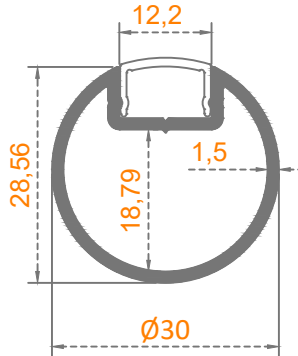
Ø 30'LUK DİKME
