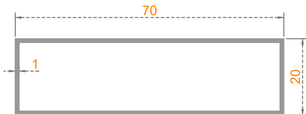
Sistem Kodu: 20-160 Ağırlık (kg/mt) 0,480
