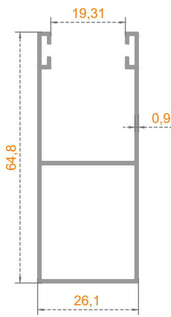
Sistem Kodu: 38-1243 Ağırlık (kg/mt) 0,480
