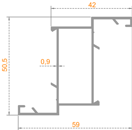
KANAT
