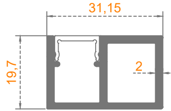
Sistem Kodu: 58-2267 Ağırlık (kg/mt) 0,515
