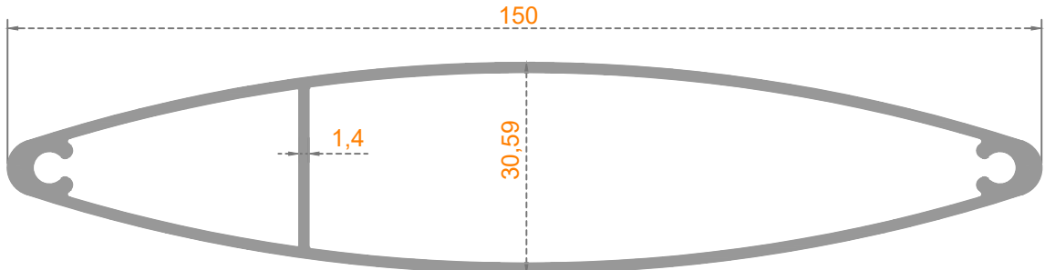
GÜNEŞ KIRICI
