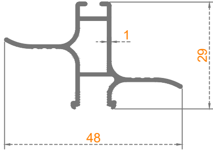
KANAT ÇEKME
