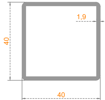
Sistem Kodu: 20-134 Ağırlık (kg/mt) 0,773
