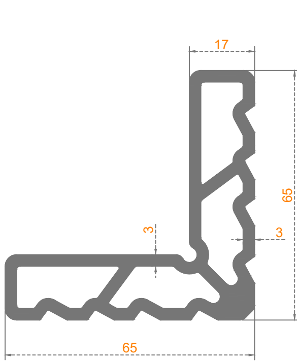
S.ÇERÇEVE TAKOZU
