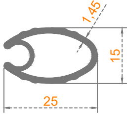
Sistem Kodu: 57-2518 Ağırlık (kg/mt) 0,275
