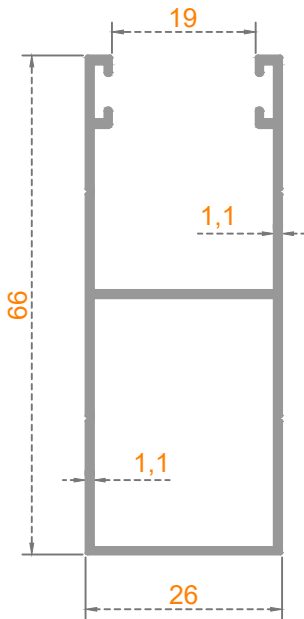
Sistem Kodu: 38-1237 Ağırlık (kg/mt) 0,575
