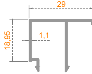
TEK CAM ÇITASI
