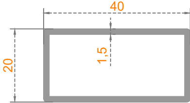
Sistem Kodu: 20-213 Ağırlık (kg/mt) 0,465
