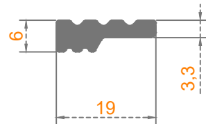
Sistem Kodu: 80-5071 Ağırlık (kg/mt) 0,210
