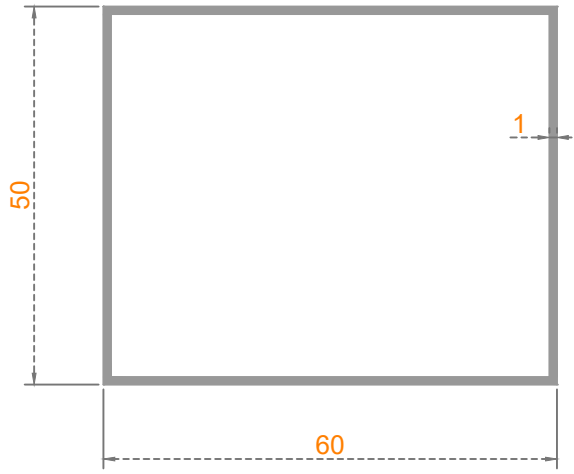
Sistem Kodu: 20-147 Ağırlık (kg/mt) 0,590
