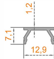
Sistem Kodu: 58-2400 Ağırlık (kg/mt) 0,081
