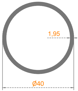
Ø 40'LUK BORU
