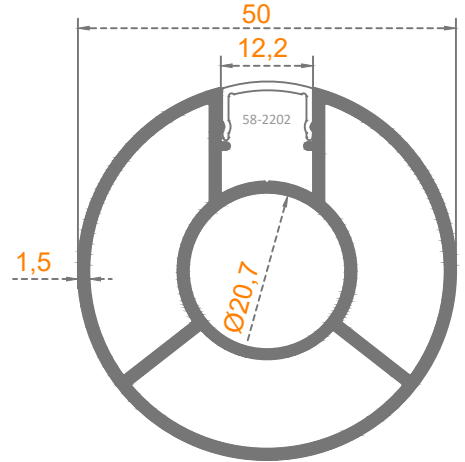
Ø 50'LUK DİKME
