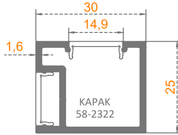
Sistem Kodu: 58-2322 Ağırlık (kg/mt) 0,430
