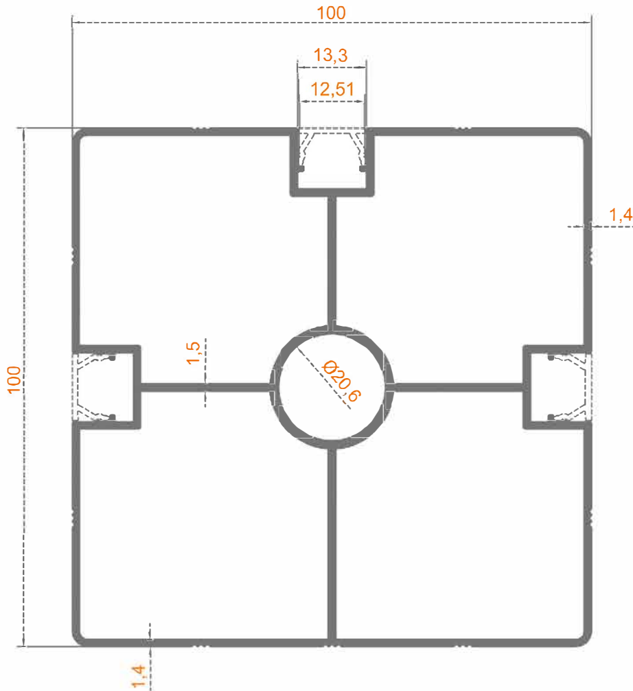
Sistem Kodu: 58-2403 Ağırlık (kg/mt) 2,521
