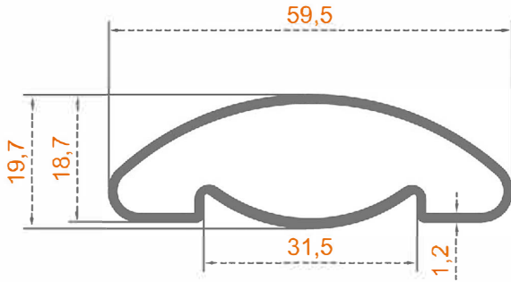
Sistem Kodu: 58-2399 Ağırlık (kg/mt) 0,475
