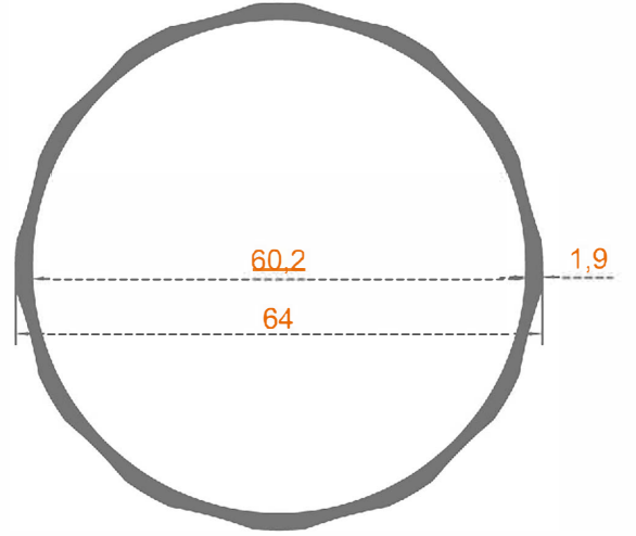
Sistem Kodu: 58-2404 Ağırlık (kg/mt) 0,849
