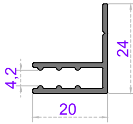
Sistem Kodu 62-1718 Ağırlık (kg/mt) 0,230
