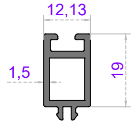
Sistem Kodu 50-1608 Ağırlık (kg/mt) 0,285
