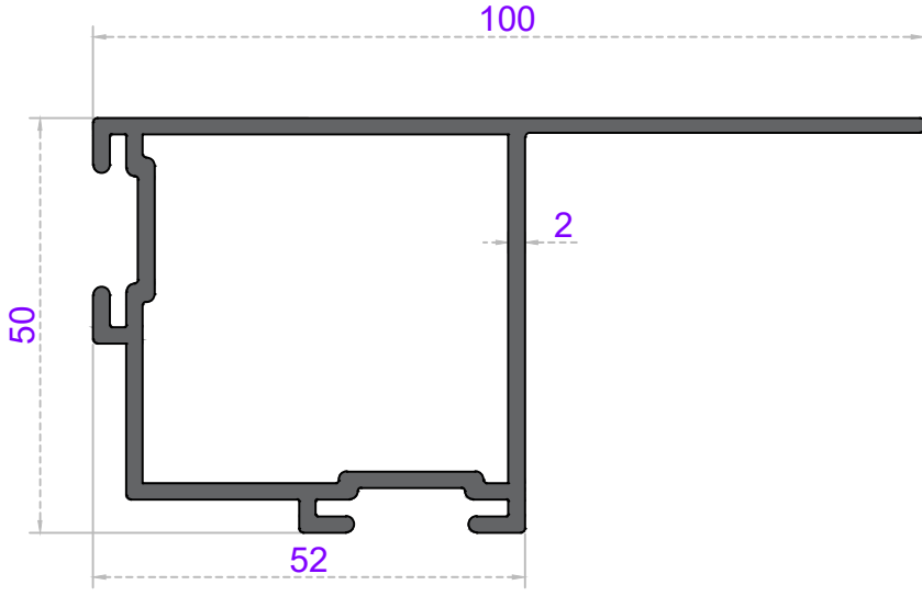
Sistem Kodu 50-1671 Ağırlık (kg/mt) 1,440
