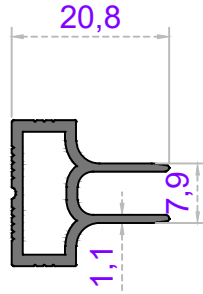
Sistem Kodu 50-1607 Ağırlık (kg/mt) 0,270
