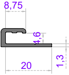
Sistem Kodu 50-1480 Ağırlık (kg/mt) 0,152
