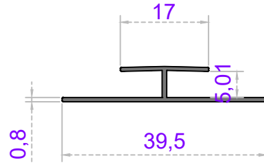
Sistem Kodu 50-1484 Ağırlık (kg/mt) 0,135
