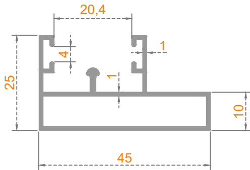
Sistem Kodu: 45-1436 Ağırlık (kg/mt) 0,455
