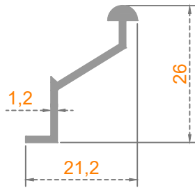
Sistem Kodu: 45-1433 Ağırlık (kg/mt) 0,152
