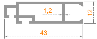
Sistem Kodu: 45-1435 Ağırlık (kg/mt) 0,377
