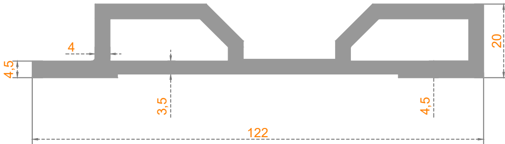
İSKELE PROFİLLER
