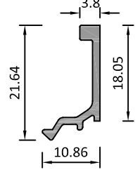
24 mm Cam Çıtası
