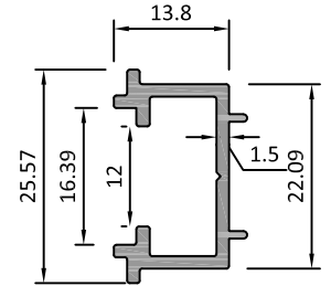
PVC İspanyolet Kanalı
