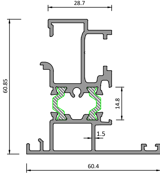
ÇİFT KANAT ADAPTÖRÜ (PVC LEVYE KOL AKSESUARLI)
