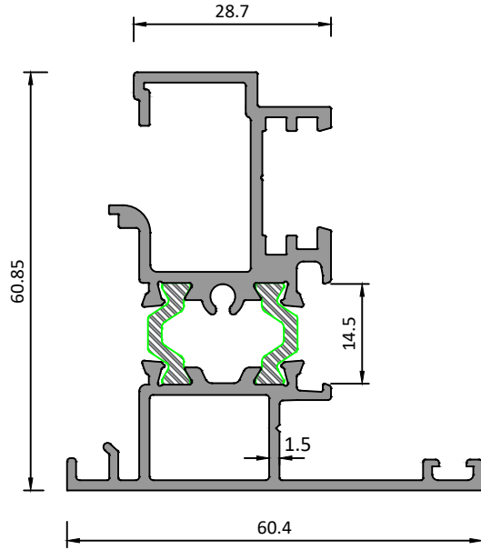
ÇİFT KANAT ADAPTÖRÜ (ALÜMİNYUM LEVYE KOL AKSESUARLI)
