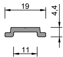
Sistem Kodu 70 - 3025 Ağırlık (kg/mt) 0,125
