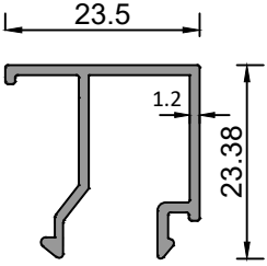
Sistem Kodu 75-10012 Ağırlık (kg/mt) 0,250
