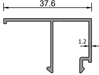
Sistem Kodu 75-10020 Ağırlık (kg/mt) 0,283
