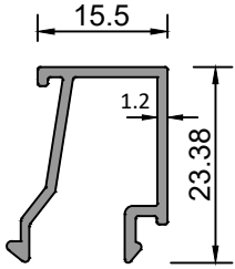
Sistem Kodu 75-10016 Ağırlık (kg/mt) 0,224
