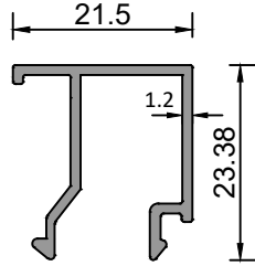
Sistem Kodu 75-10013 Ağırlık (kg/mt) 0,243
