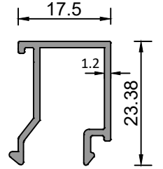
Sistem Kodu 75-10015 Ağırlık (kg/mt) 0,230
