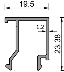
Sistem Kodu 75-10014 Ağırlık (kg/mt) 0,237
