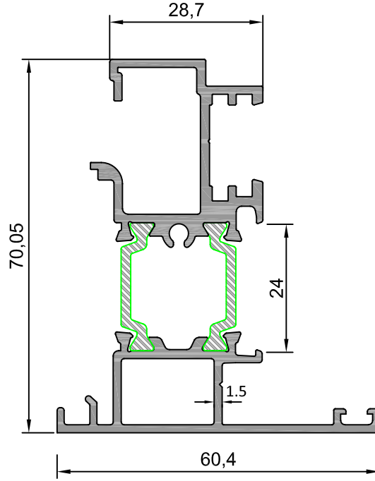
ÇİFT KANAT ADAPTÖRÜ (ALÜMİNYUM LEVYE KOL AKSESUARLI)
