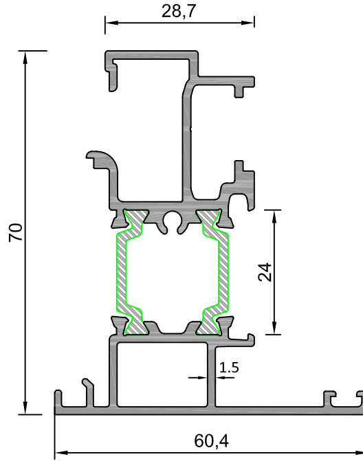
ÇİFT KANAT ADAPTÖRÜ (PVC LEVYE KOL AKSESUARLI)
