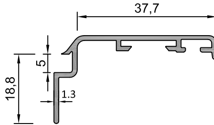
Sistem Kodu 35-10836 Ağırlık (kg/mt) 0,298
