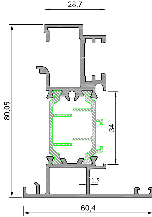
ÇİFT KANAT ADAPTÖRÜ (ALÜMİNYUM LEVYE KOL AKSESUARLI)
