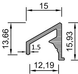
Sistem Kodu 70-10224 Ağırlık (kg/mt) 0.183
