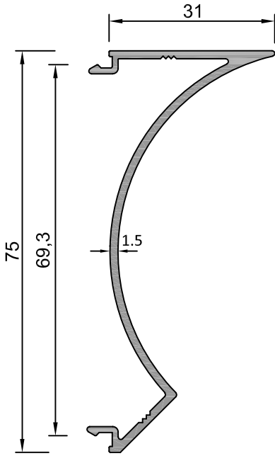
Sistem Kodu 70-10422 Ağırlık (kg/mt) 0,550
