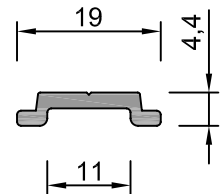
Sistem Kodu 70 - 3025 Ağırlık (kg/mt) 0.125
