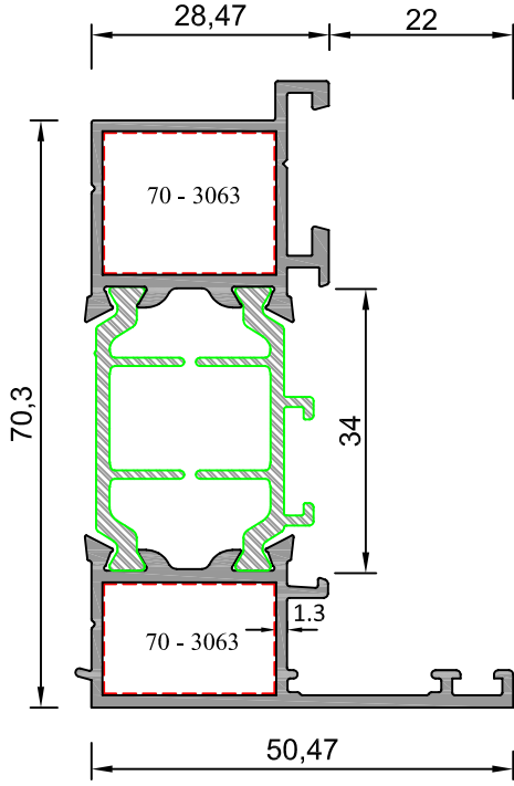
DIŞA AÇILIR KANAT ADAPTÖRÜ
