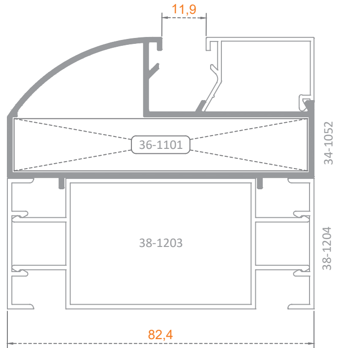
MONTAJ DETAYI
