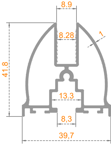
Sistem Kodu: 41-2718 Ağırlık (kg/mt) 0,665
