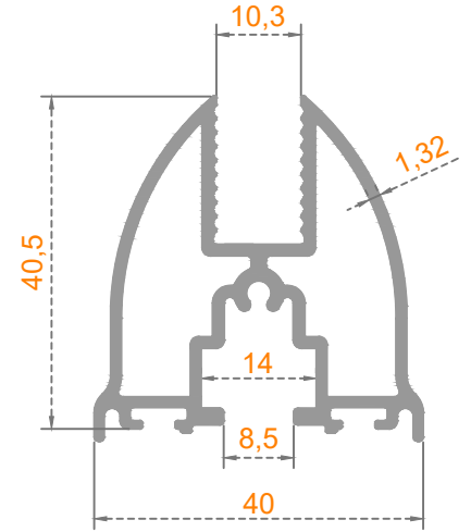
Sistem Kodu: 41-2716 Ağırlık (kg/mt) 0,848
