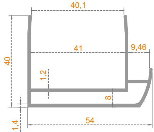
Sistem Kodu: 41-2481 Ağırlık (kg/mt) 0,635
