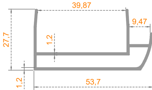
Sistem Kodu: 41-2480 Ağırlık (kg/mt) 0,518
