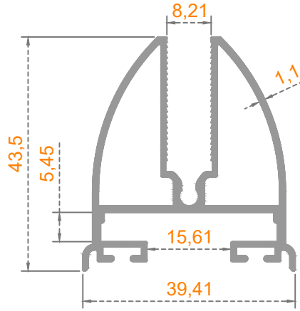
Sistem Kodu: 41-2843 Ağırlık (kg/mt) 0,700
