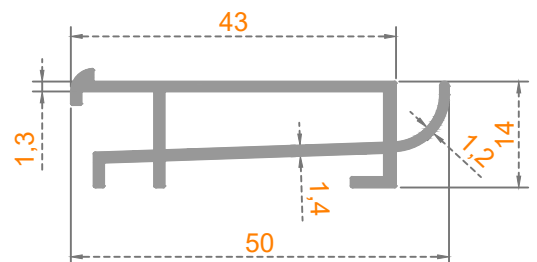
Sistem Kodu: 41-2703 Ağırlık (kg/mt) 0,480
