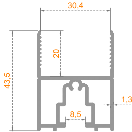
Sistem Kodu: 41-2829 Ağırlık (kg/mt) 0,679
